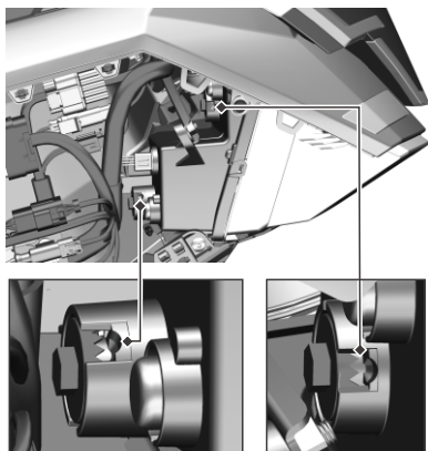
近光灯调节
