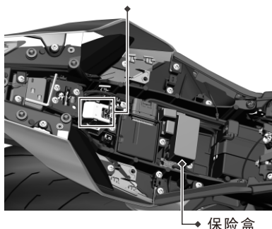
启动继电器
