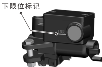
前碟刹主泵
