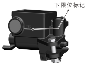
后碟刹主泵
