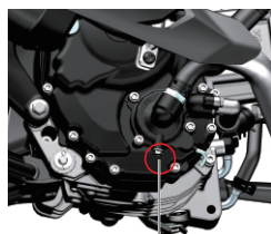
放水螺栓
