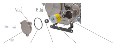
精滤器盖 密封O圈 精滤器弹簧 机油精滤器 机油精滤器密封圈
