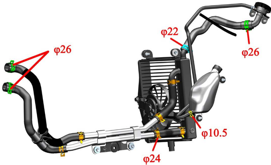
冷却液系统抱箍/卡箍分布图
