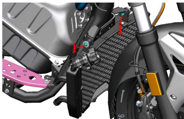
冷却液系统抱箍/卡箍分布图
