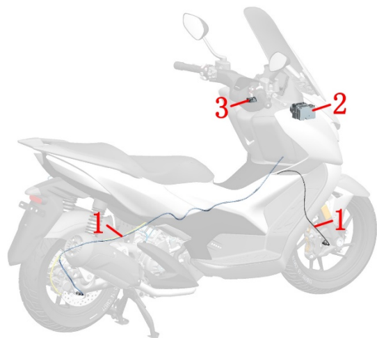
1-前、后轮轮速传感器 2-ABS 液控单元 3-OBD 诊断接口 ABS 液控单元
