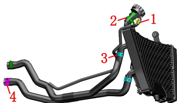
冷却液系统抱箍/卡箍分布图
