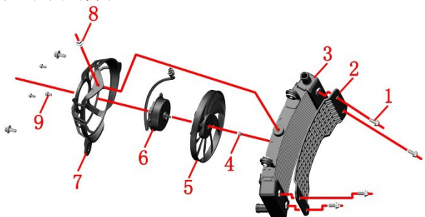
1-水箱前护罩螺栓*4 2-水箱前护罩 3-水箱 4-扇页 5-扇页 6-风扇电机
