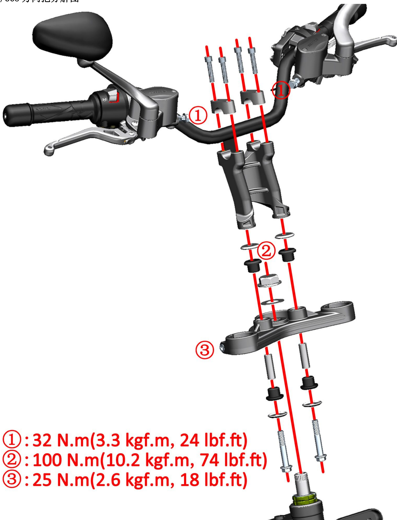
M350/368 方向把分解图
