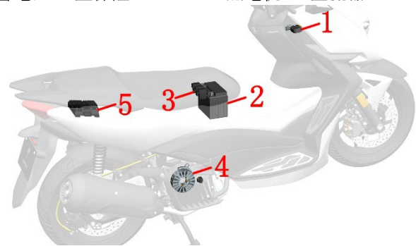
1-充电口（PKE） 2-蓄电池 3-主保险（25A） 4-磁电机 5-启停控制器（M150）
