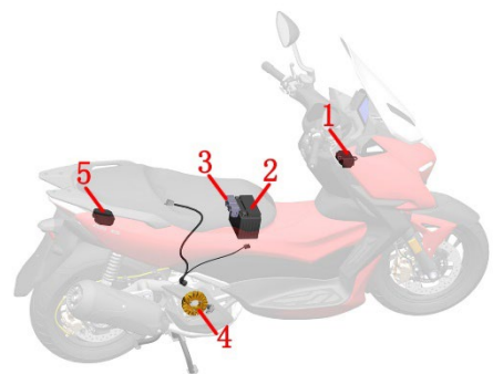
1-充电口（PKE） 2-蓄电池 3-主保险（25A） 4-磁电机 5-整流器（M310/350/368/368 ETC）
