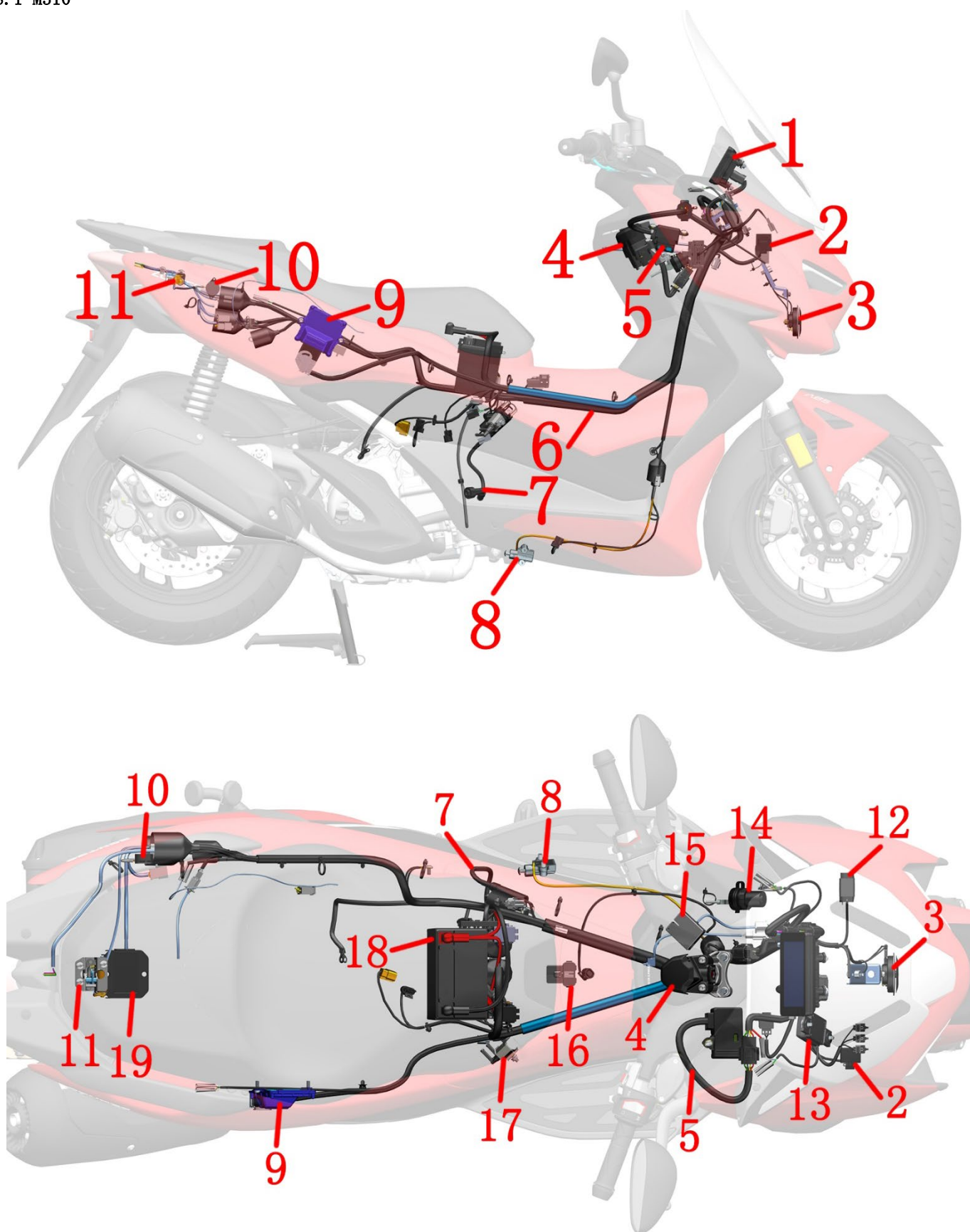
1-TFT 仪表 2-闪光器 3-喇叭 4-龙头锁 5-PKE 6-主电缆 7-点火线圈 8-侧支架熄火开关 9-发动机控制器 (ECU) 10-蜂鸣器 11-坐垫锁 12-倾倒开关 13-风挡电机控制器 14-USB 充电线 15-前储物箱锁 16-电子油箱锁 17-碳罐电磁阀 18-蓄电池 19-整流器
