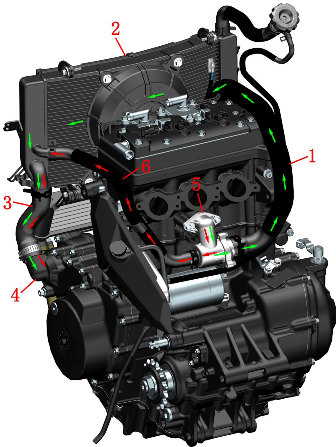
冷却液流动示意图
