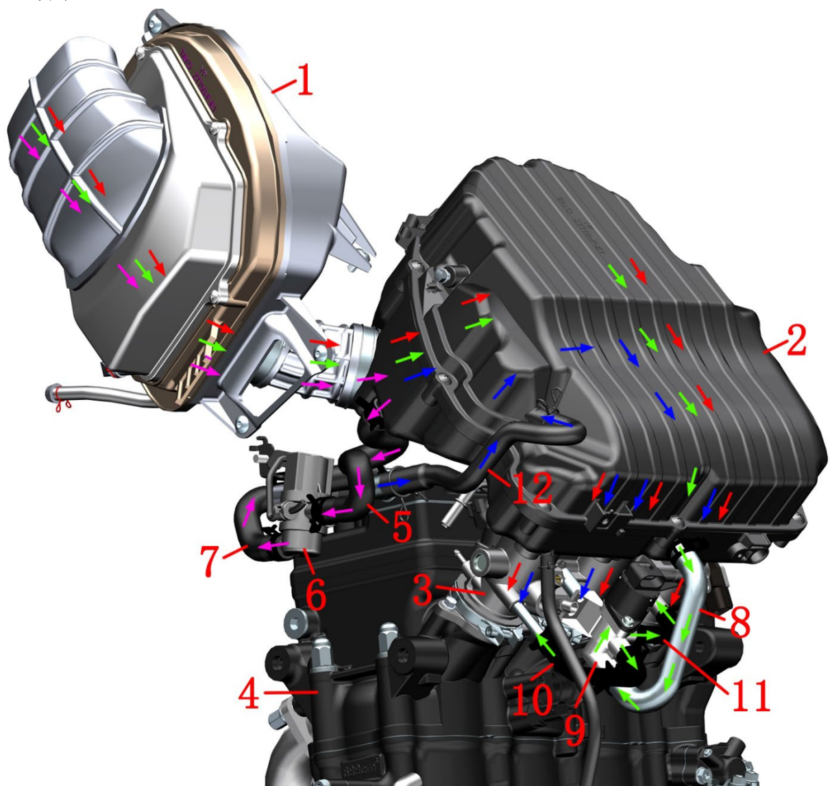
1-左侧进气腔体组件 2-空滤器组件 3-节气门阀体组件 4-缸头 5-补气阀橡胶管-4 6-补气阀 7-补气阀橡胶管 -3 8-步进电机橡胶管-2 9-节气门补气阀 10-步进电机橡胶管-1 11-步进电机橡胶管-3 12-废气通气管
