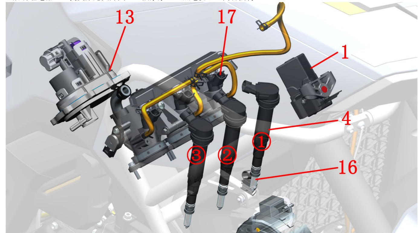
16-火花塞 17-喷油嘴
