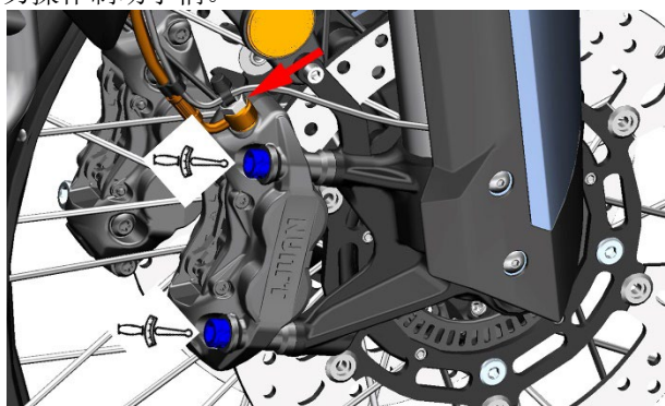
前碟刹卡钳分解
