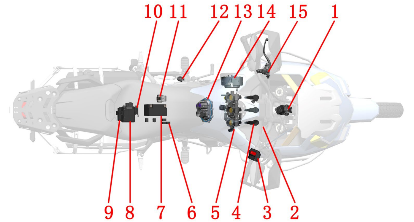
电喷零件布局图
