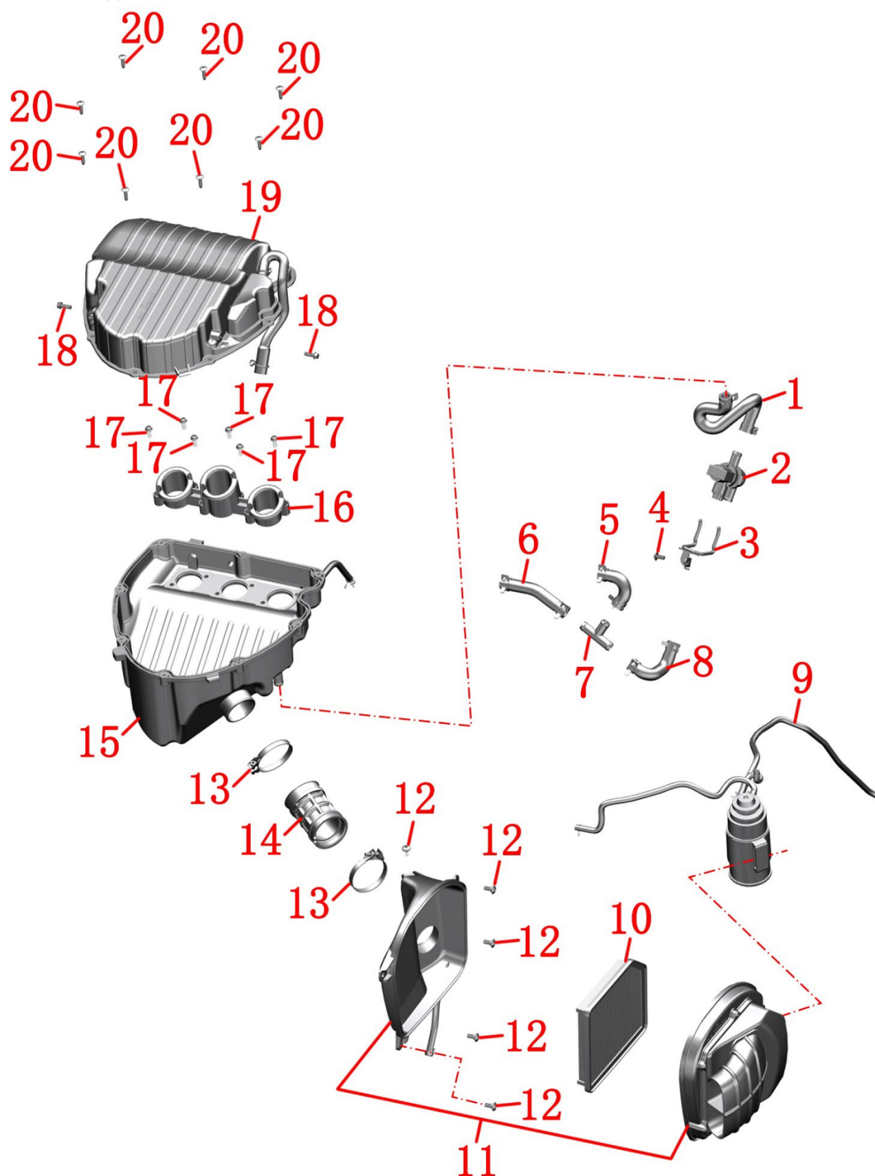
空滤器组件分解图
