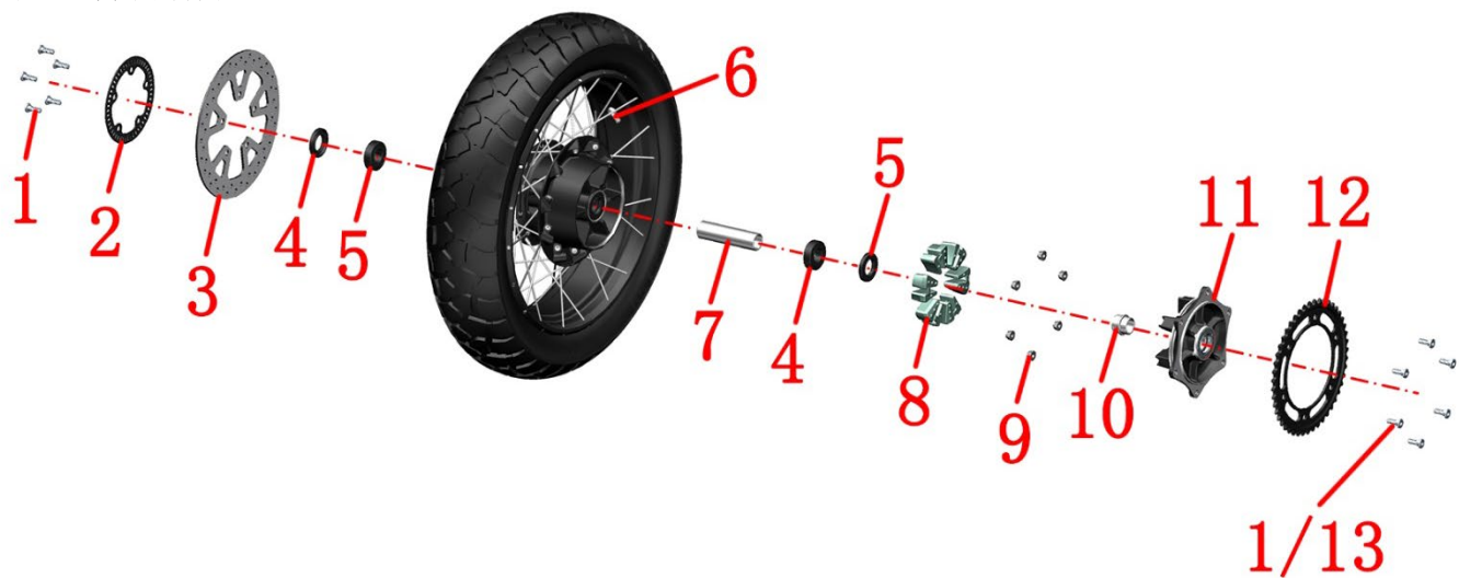
后轮组件分解图：
