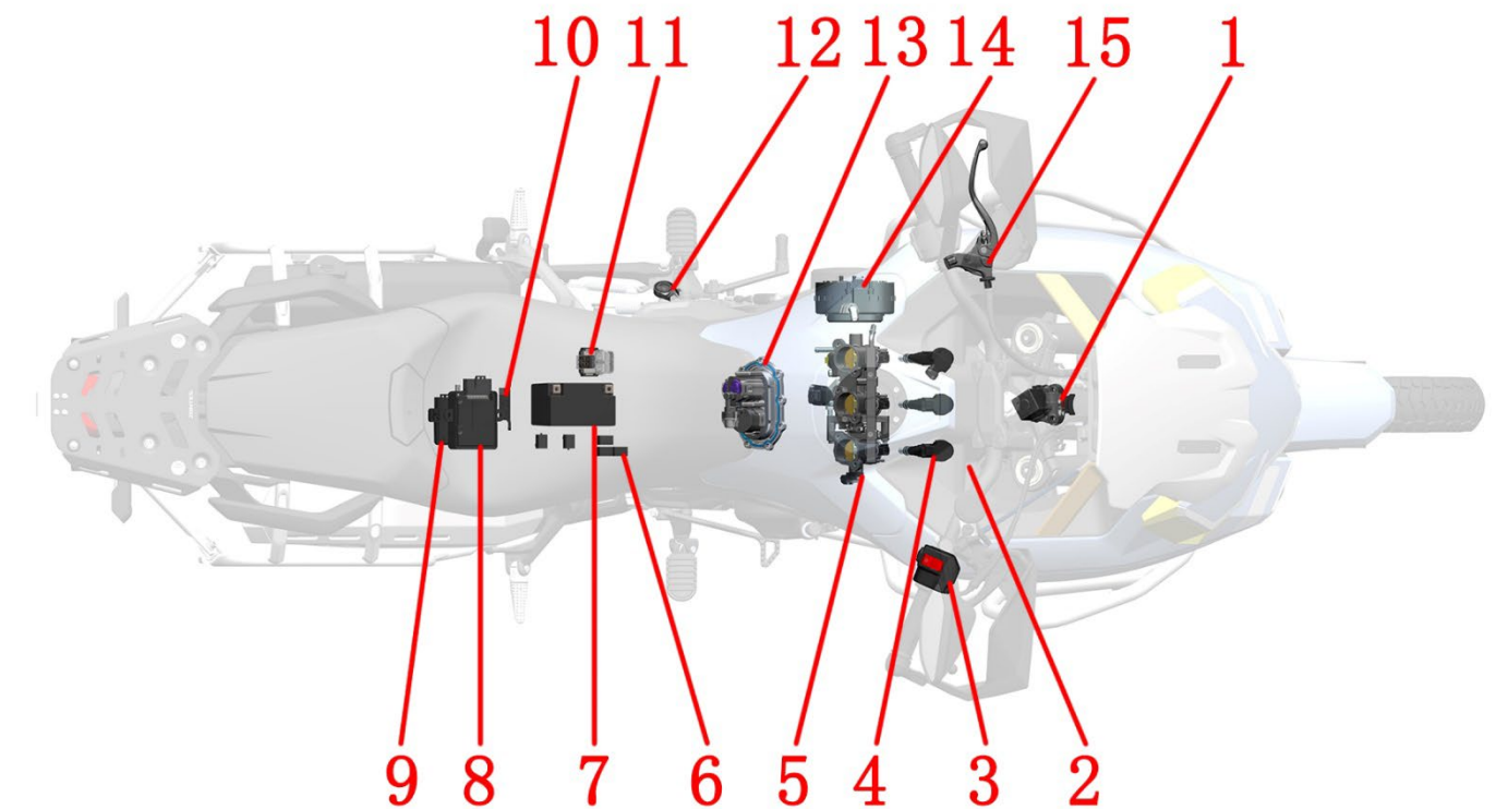
1-龙头锁 2-氧传感器 3-右手把开关 4-点火线圈 5-节气门组件 6-继电器（主线束保险盒内有 3 件，保险盒外侧有 2 件） 7-蓄电池 8-PKE 主机 9-ECU 10-倾倒开关 11-启动继电器 12-侧支架熄火开关 13-油泵泵 14-磁电机 15-离合摇臂
