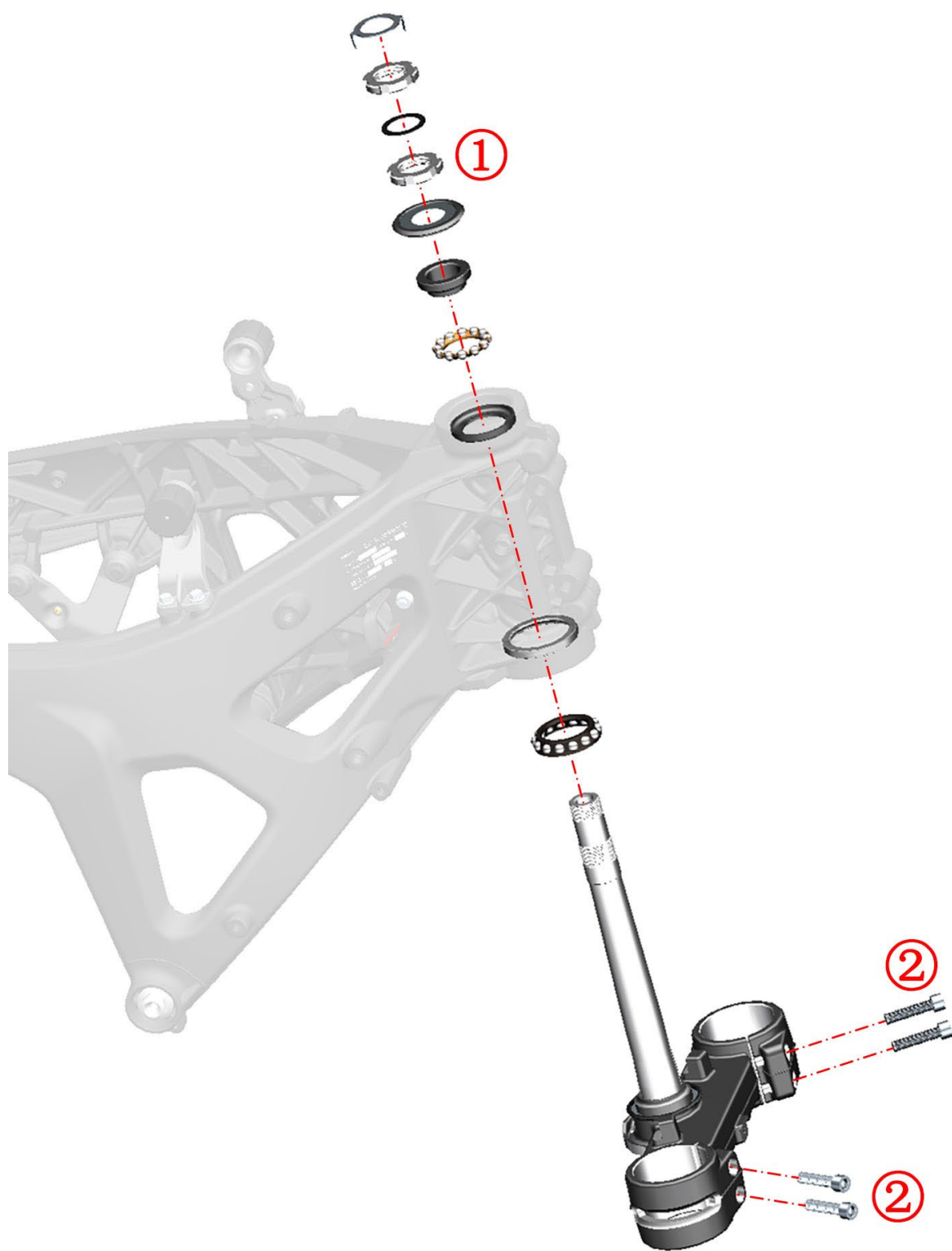
下联板分解图
