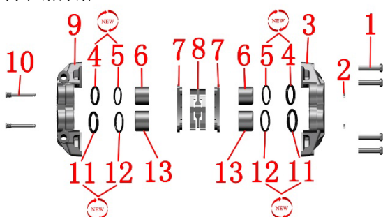
前碟刹卡钳分解
