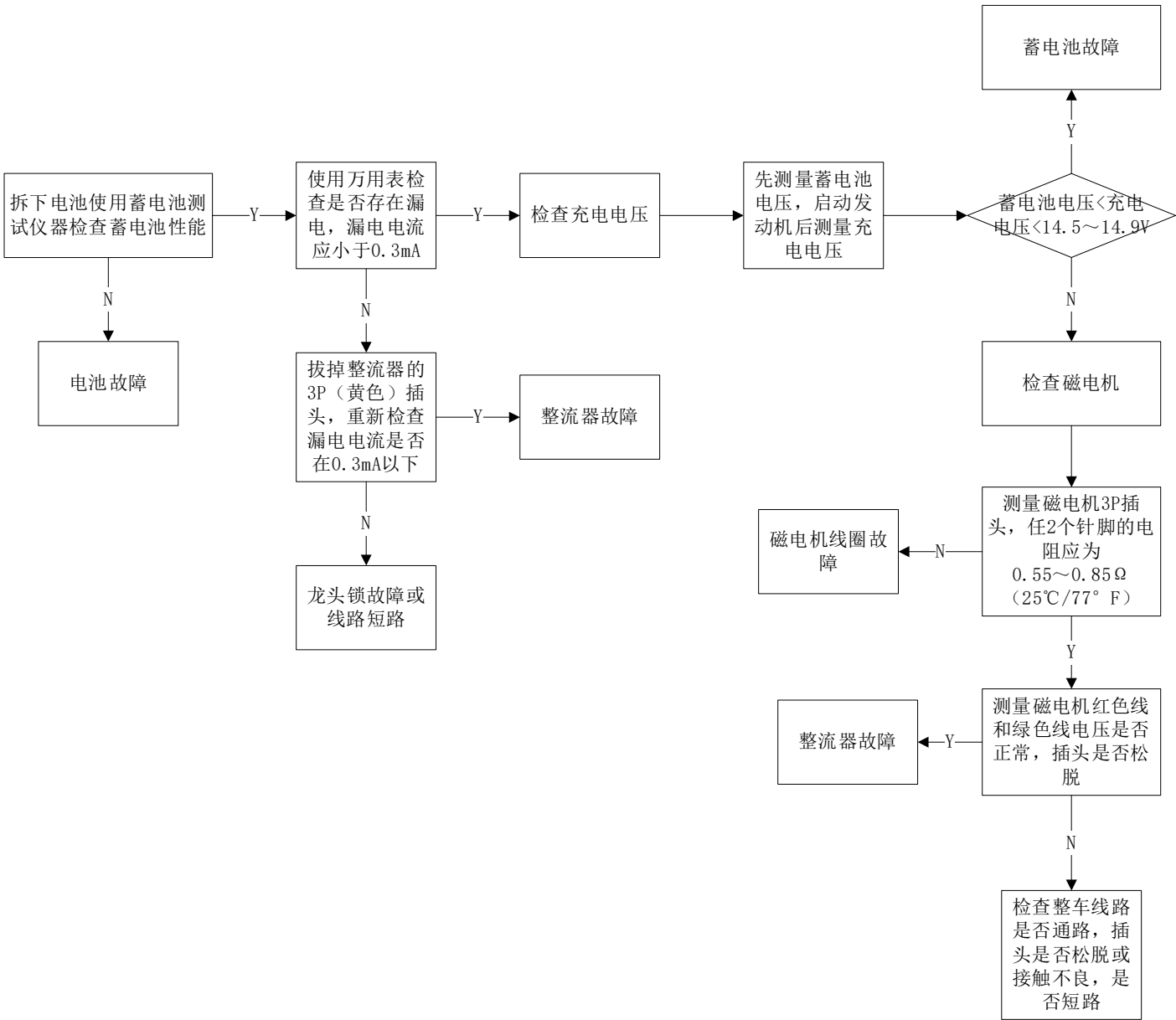
蓄电池损坏或衰减排查流程
