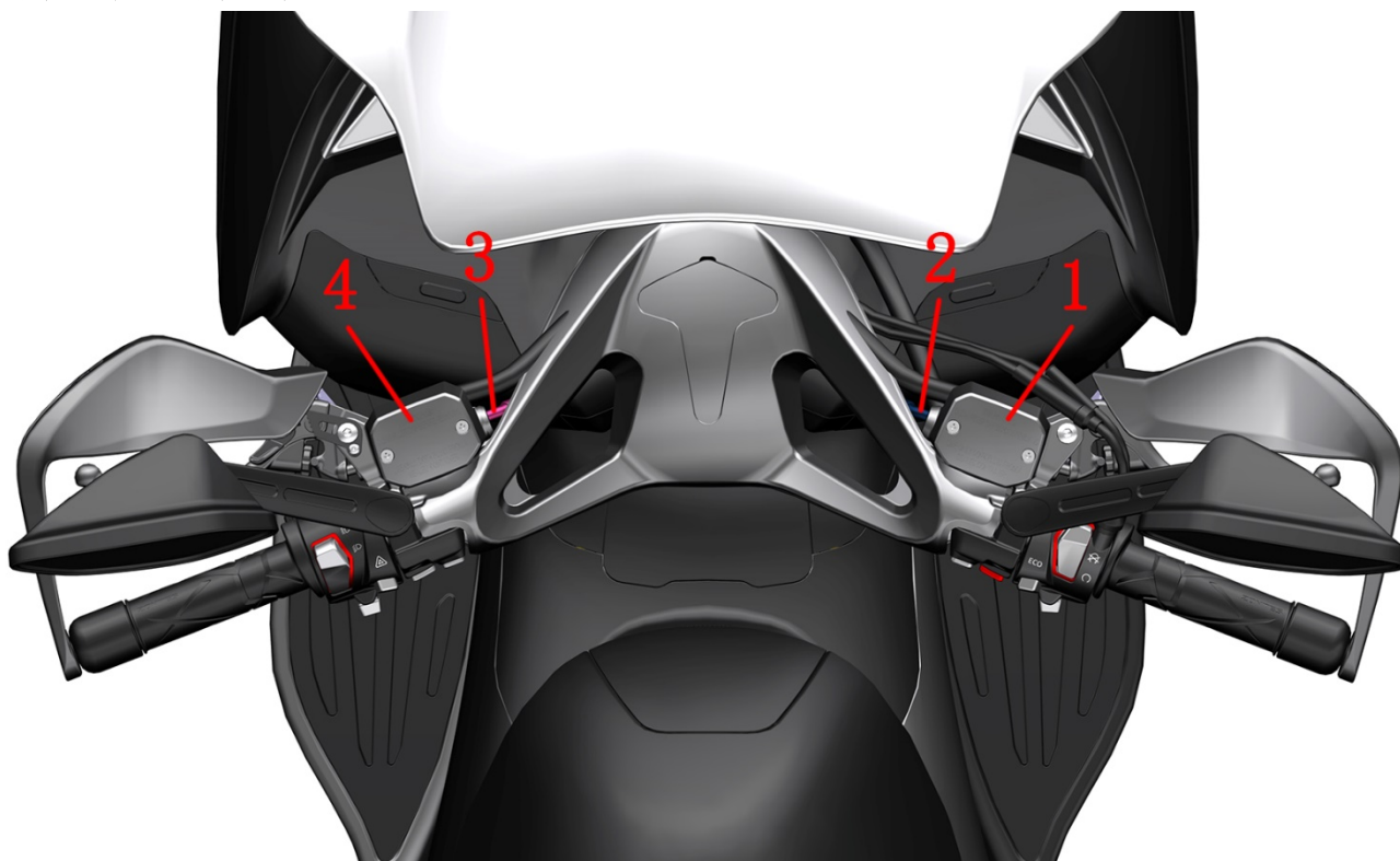
1-前碟刹主泵 2-FMC-HU 制动软管 3-RMC-HU 制动软管 4-后碟刹主泵
