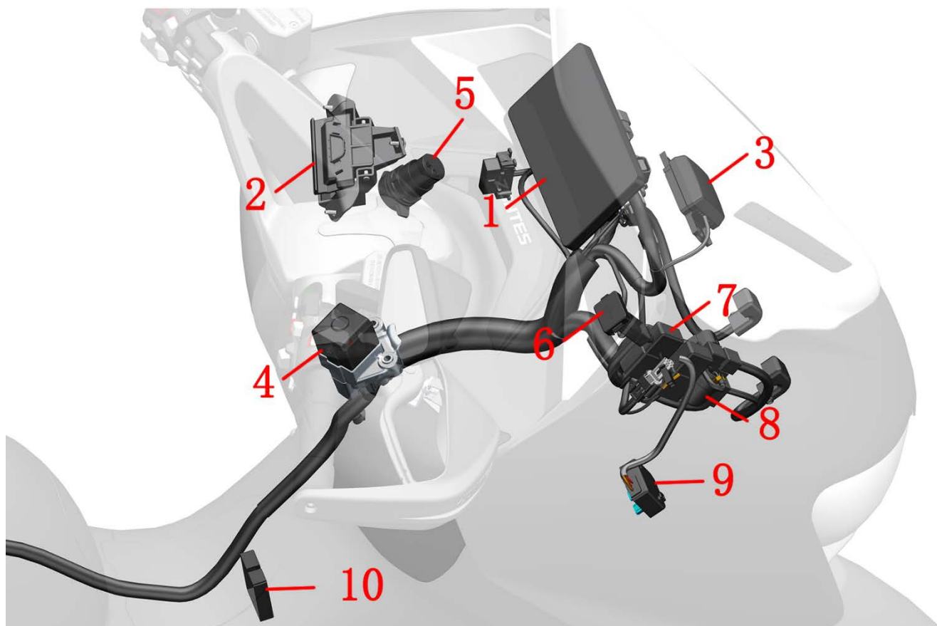
1-TFT 仪表 2-前左储物箱锁 3-风挡电机控制器 4-龙头锁 5-双口 USB 充电线 6-单口充电线 7-电喷继电器 8-启动继电器 9-充电插座 10-油箱电子锁
