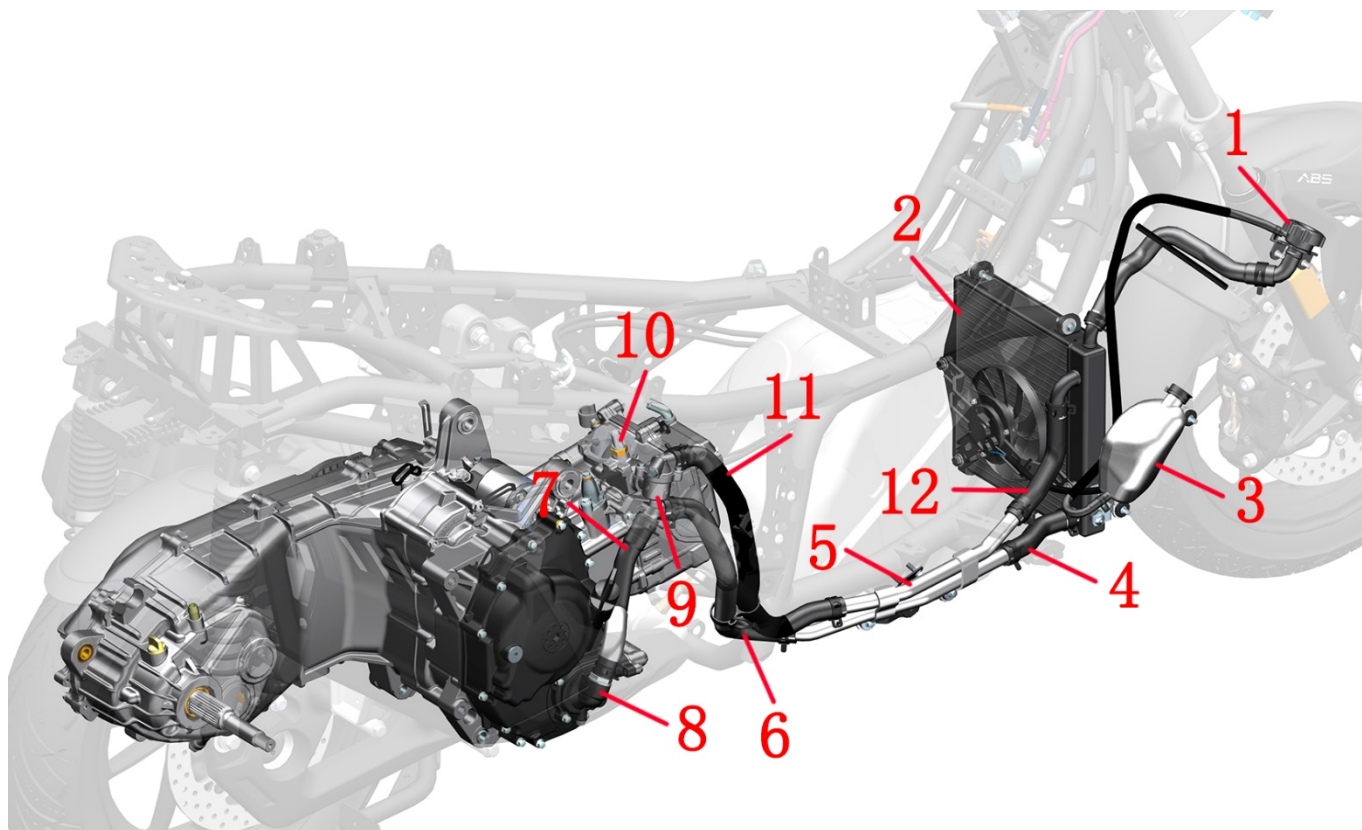
1-主水箱加注口 2-主水箱 3-副水箱 4-主水箱出水管 5-铝过水管 6-发动机过水管 7-水泵盖进水管 8-水泵盖组件 9-节温器组件 10-水油共用传感器 11-节温器出水管 12-主水箱进水管
