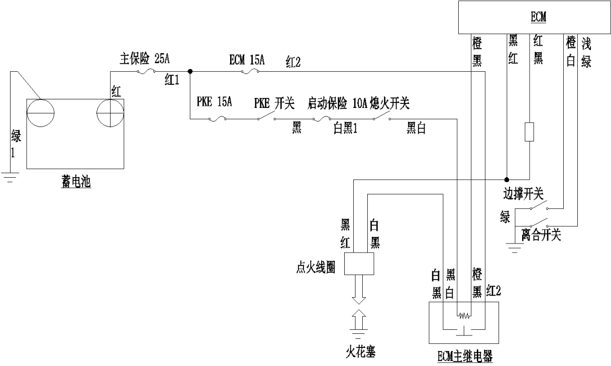
点火系统电气原理图
