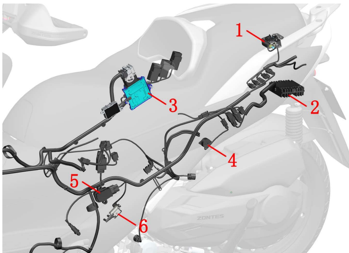
1-坐垫锁 2-整流器 3-发动机控制器（ECU） 4-蜂鸣器 5-点火线圈本体 6-碳罐电磁阀
