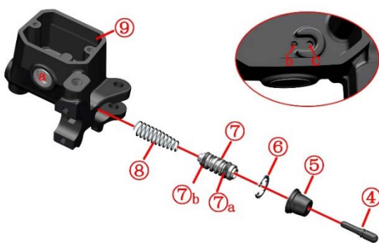
④活塞推杆 ⑤防尘帽 ⑥挡圈 ⑦活塞组件（⑦a 外密封圈 ⑦b 内密封圈） ⑧弹簧 ⑨主泵壳体
