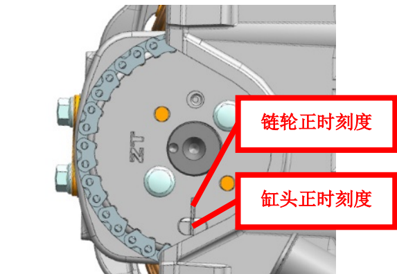
链轮正时刻度与缸头正时刻度对齐 飞轮检具：
