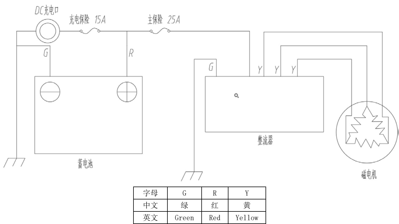
电气原理图
