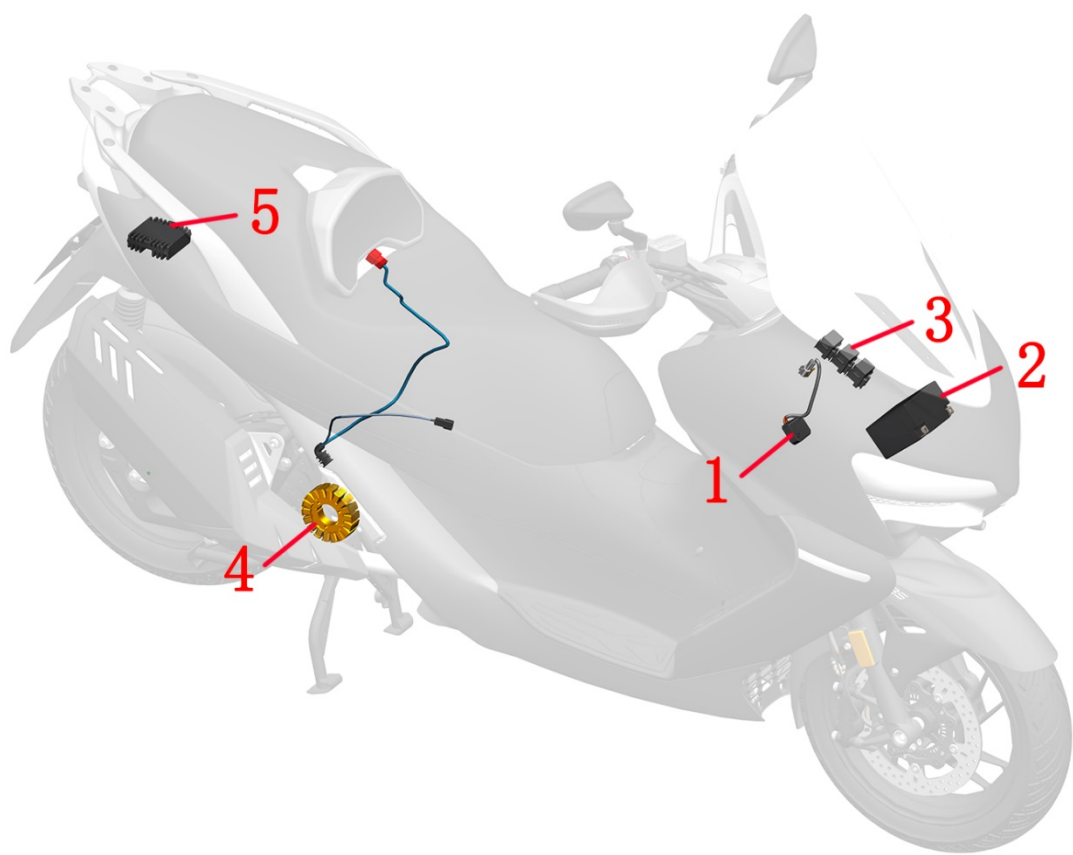
1-充电口（PKE） 2-蓄电池 3-主保险（25A） 4-磁电机 5-整流器
