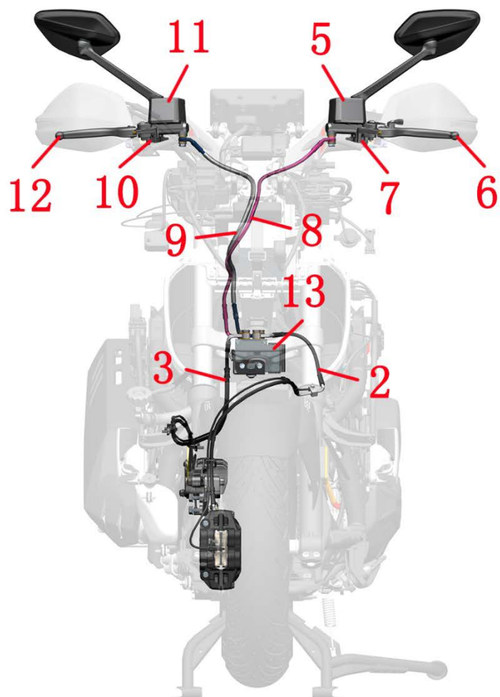
1-轮速传感器（前轮） 2-FC-HU 制动软管 3-RC-HU 制动软管 4-轮速传感器（后轮） 5-后碟刹主泵 6-后制动手柄 7-后 刹车开关 8-RMC-HU 制动软管 9-FMC-HU 制动软管 10-前刹车开关 11-前碟刹主泵 12-前制动手柄 13-液控单元
