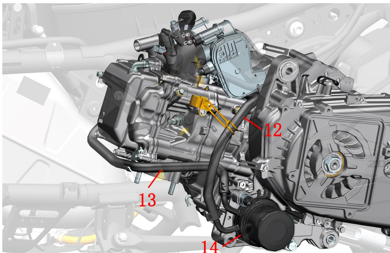
1-主水箱 2-水箱加水口 3-副水箱 4-主水箱进水管 5-主水箱出水管 6-铝过水管 7-节温器出水管 8-发动机进水管 9-水油共用传感器 10-节温器 11-水泵盖组件 12-油冷器进水管 13-油冷器出水管 14-油冷器
