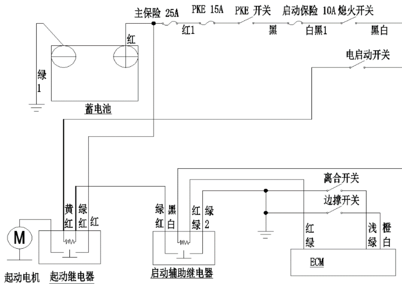
起动系统电气原理图
