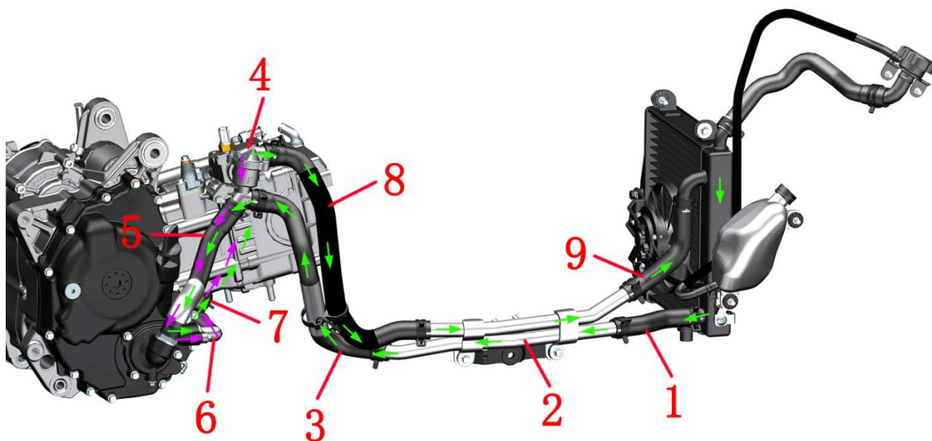
1-主水箱出水管 2-铝过水管 3-发动机过水管 4-节温器 5-水泵盖进水管 6-水泵盖出水接头 7-水泵盖出水管 8-节温器出水管 9-主水箱进水管
