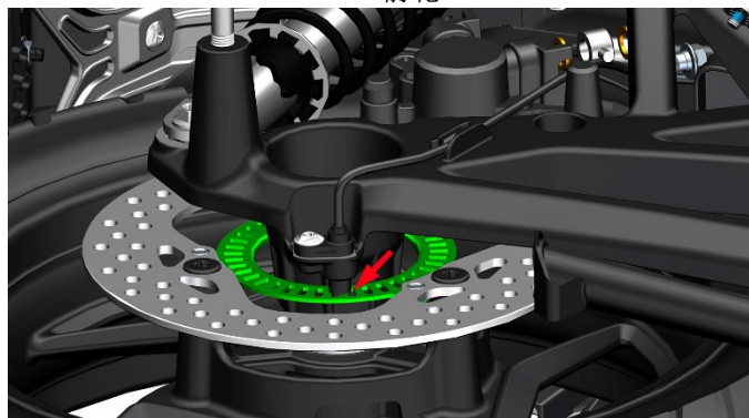
后轮
