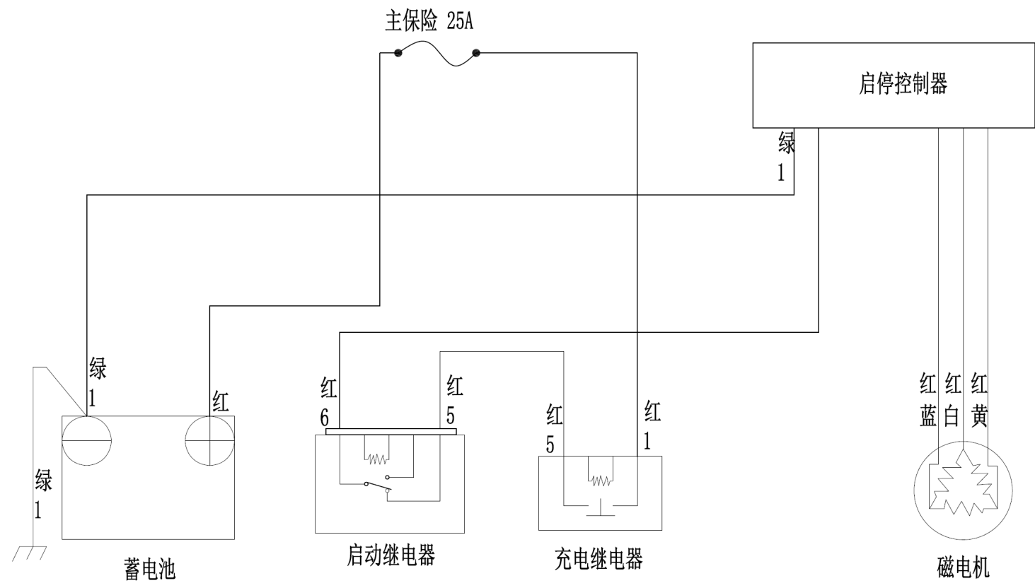
电气原理图
