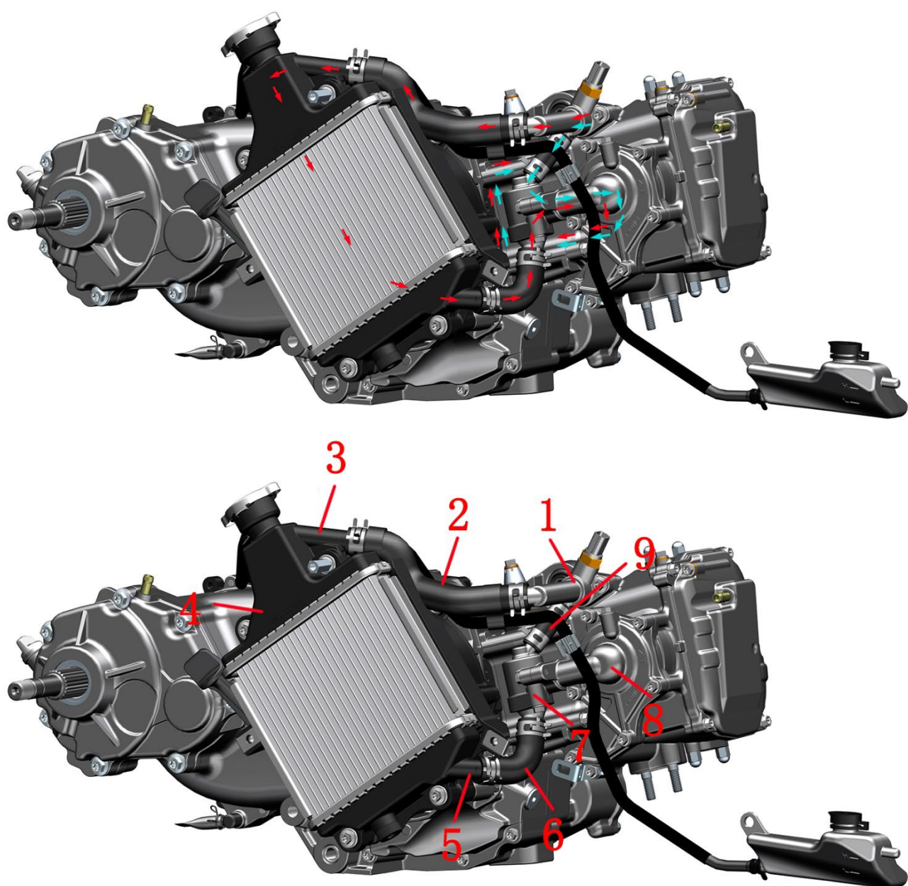
冷却液流动示意图
