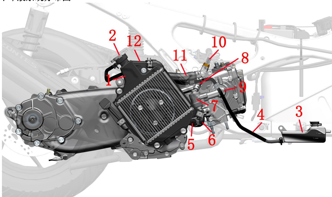
冷却液系统分布图
