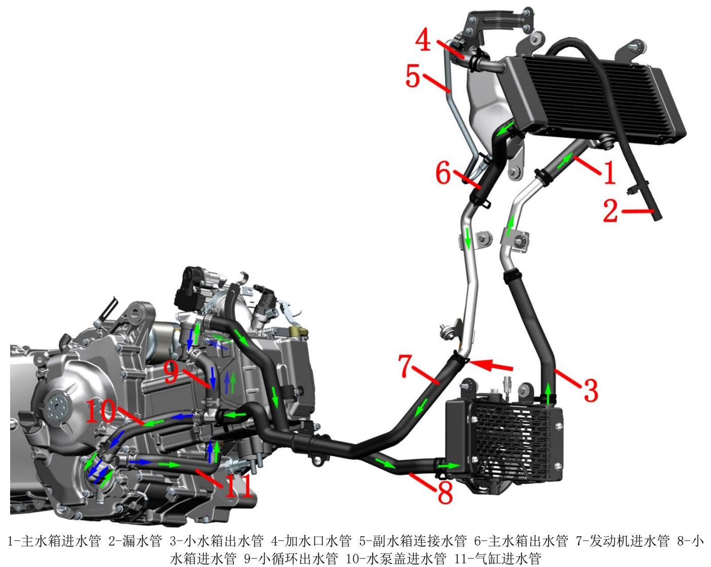
冷却液流动示意图 M310
