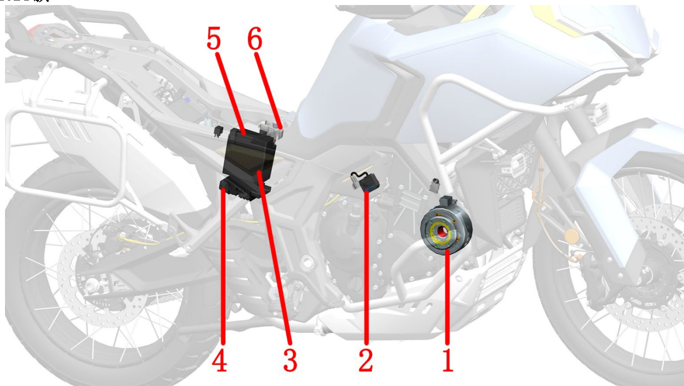
1-磁电机 2-充电口座 3-蓄电池 4-整流器 5-保险盒 6-启动继电器（40A）
