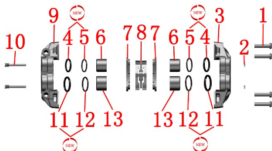
前碟刹卡钳分解
