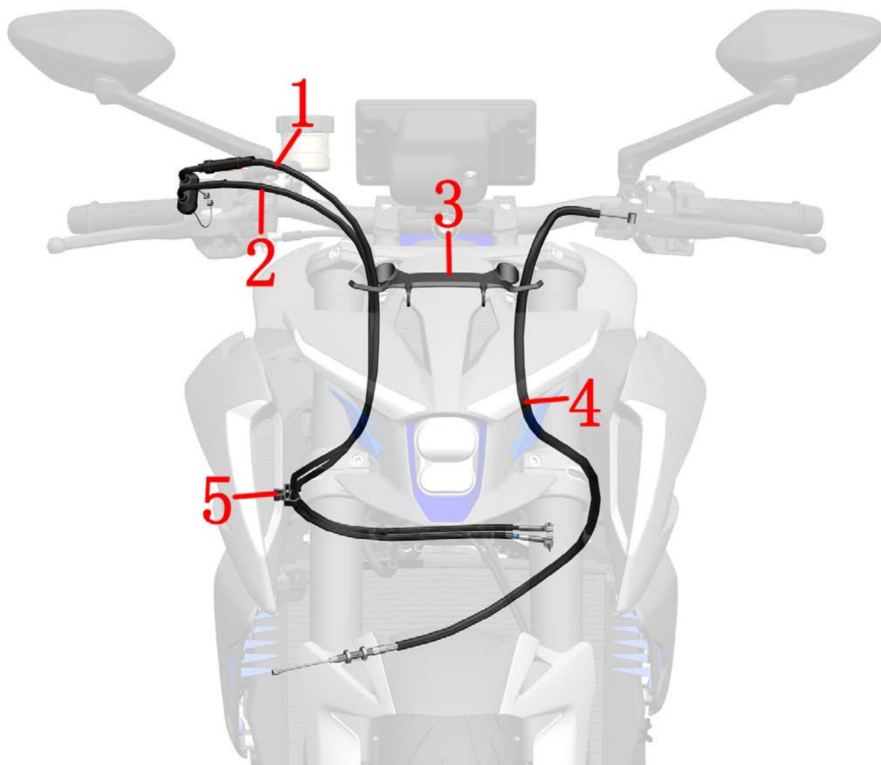
1-加油线 2-回油线 3-头部支架 4-离合线 5-油门线线夹 2026 款无加油线和回油线
