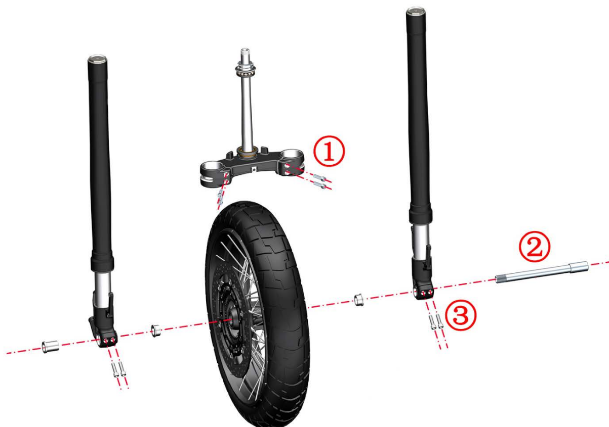
前叉分解图
