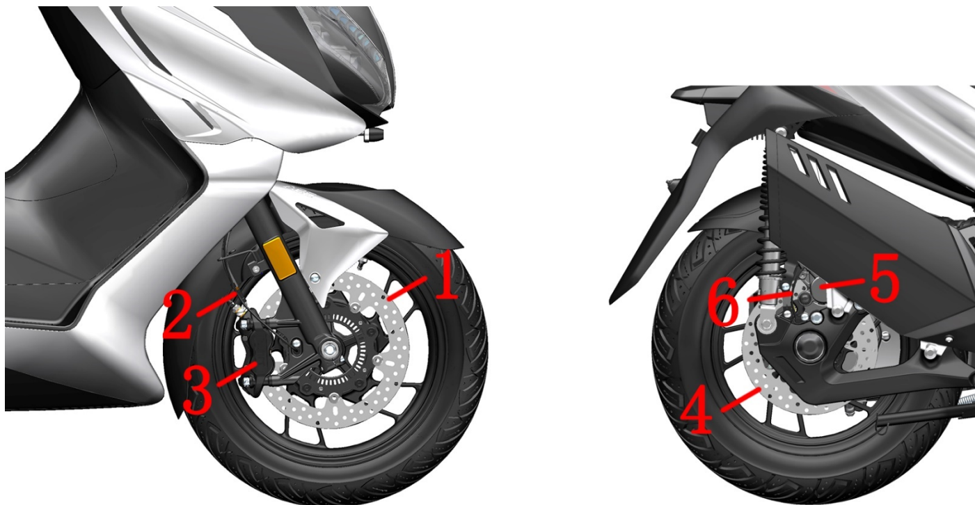
1-前制动盘组件 2-轮速传感器（前轮） 3-前碟刹卡钳 4-后制动盘组件 5-后碟刹卡钳 6-轮速传感器（后轮） E368 (ETC)
