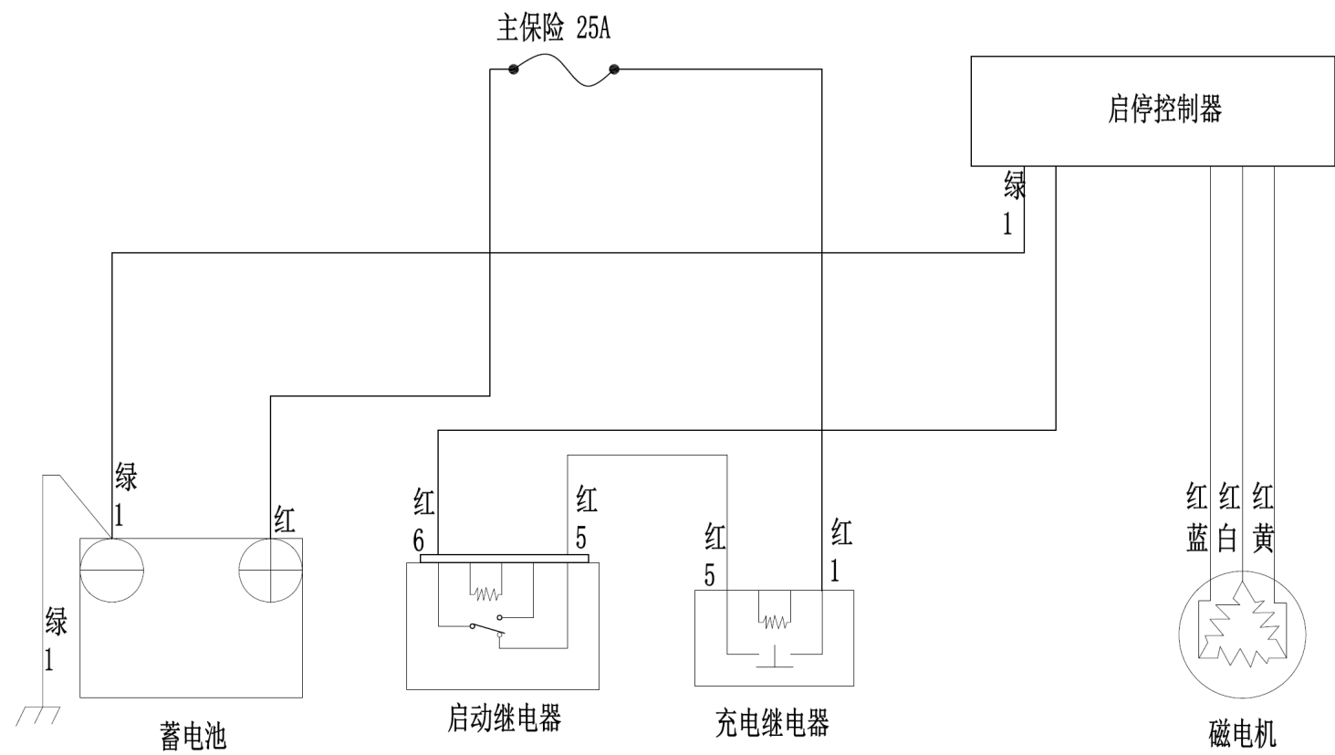
电气原理图
