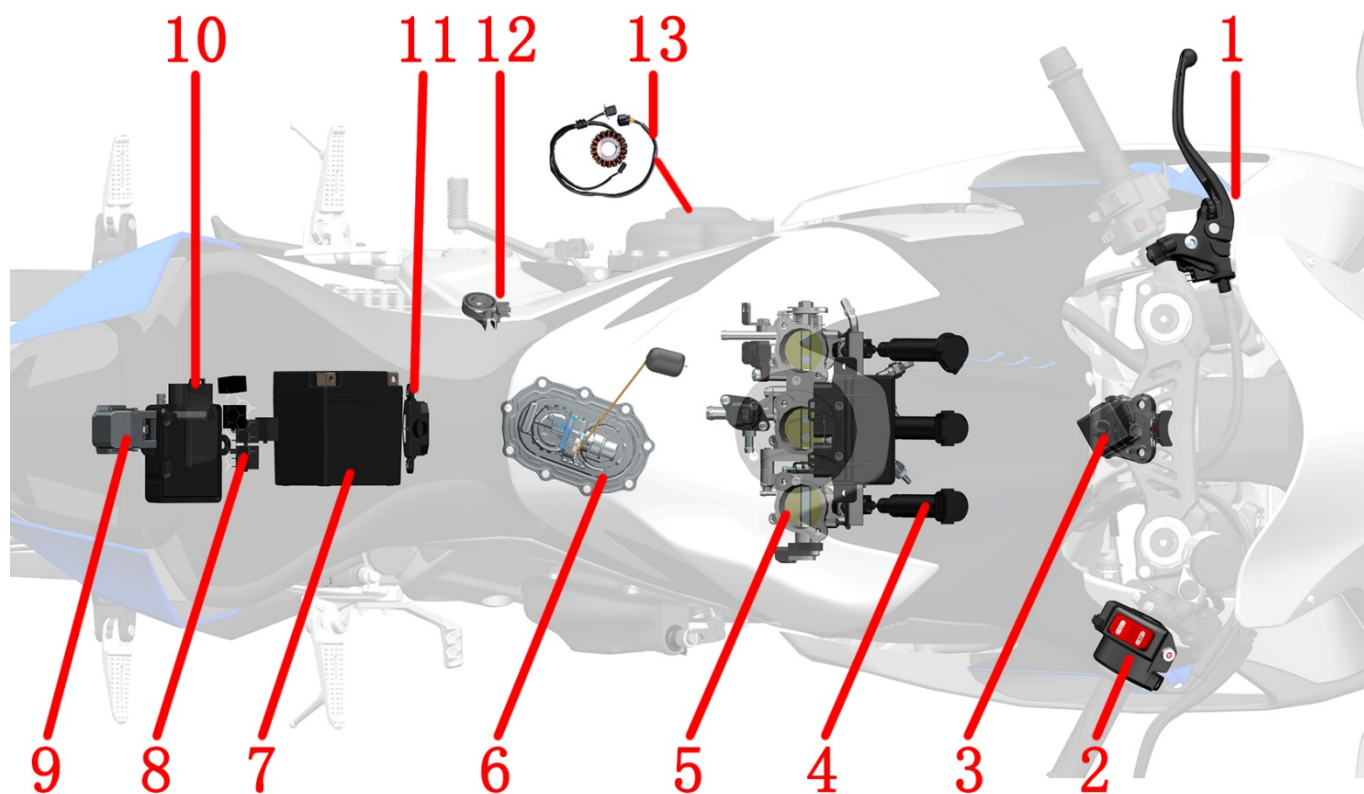
电喷零件布局图
