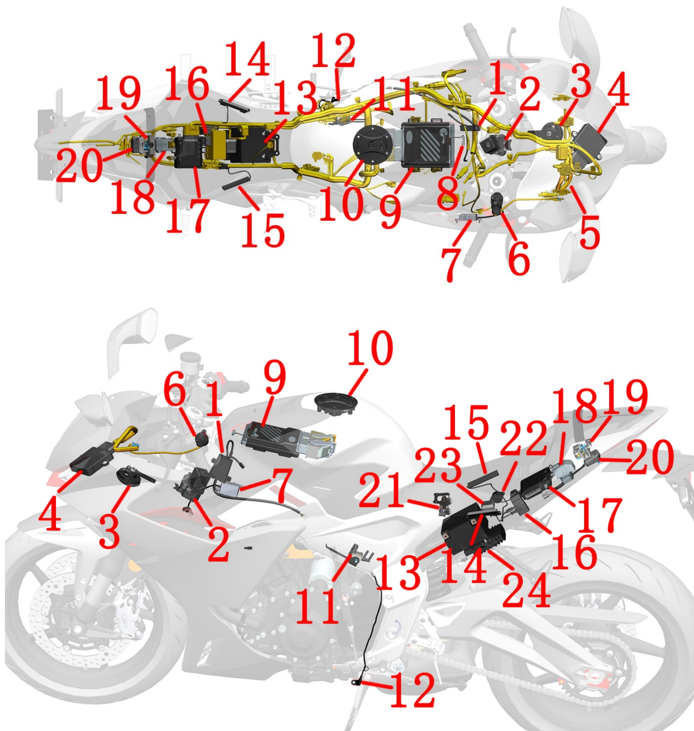
1-车架网格氛围灯驱动器 2-龙头锁 3-喇叭 4- LCM 灯光控制器 5-线缆总成（黄色所示）6-双口通用 USB 充电线 7-胎压接收主机 8-电子油箱锁基板 9-发动机控制器（ECU）10-电子油箱锁 11-碳罐电磁阀 12--侧熄火开关 13-锂电池 14-无电感应天线 15- PKE 外置天线 16-继电器 17-三代 PKE 主机 18-启动继电器 19-电子坐垫锁 20-充电口座（2026 款取消，可从 6-双口通用 USB 充电线处充电） 21-倾倒开关 22-蜂鸣器 23- GPS 天线 24-整流器
