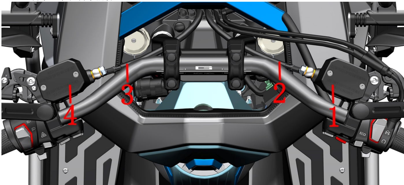
1-前碟刹主泵 2-FMC-HU 制动软管 3-RMC-HU 制动软管 4-后碟刹主泵
