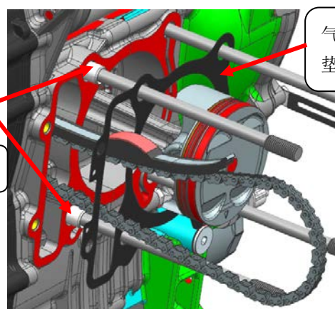
结合面涂抹密封胶
