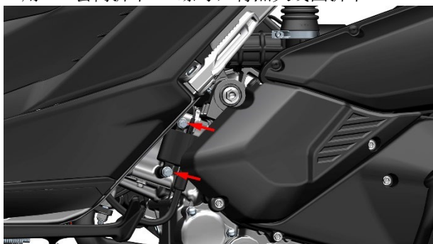
用 10#套筒拆下 M6 螺母，将点火线圈拆下。
