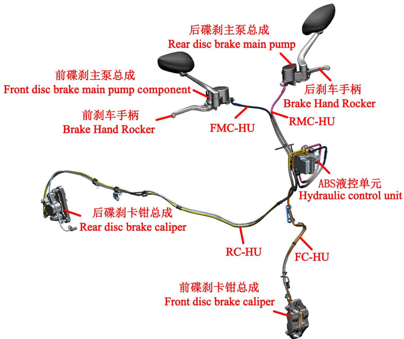
D350 制动系统部件图
