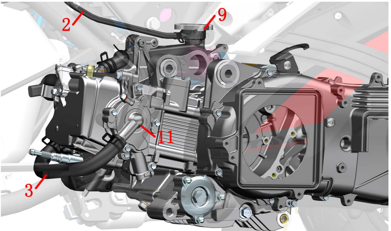
1-副水箱 2-副水箱连接水管 3-发动机进水管 4-节温器水管 5-节温器 6-水箱进水管 7-水油共用传感器 8-水箱出水管 9-水箱盖 10-散热器散件 11-水泵盖组件
