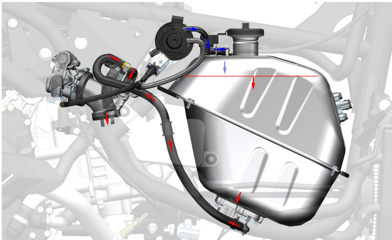
6.6 D368 燃油供应
