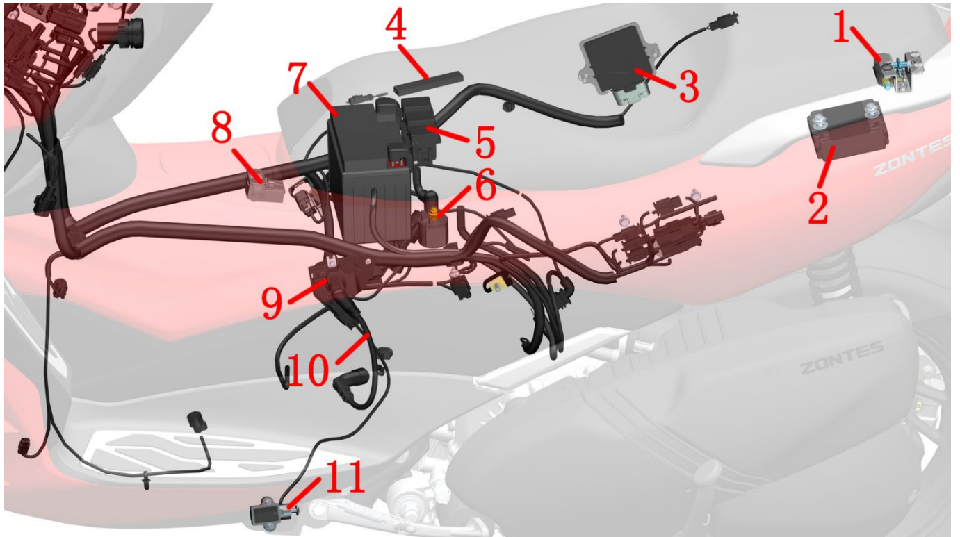
1-坐垫锁 2-整流器 3-发动机控制器 (ECU) 4-PKE 天线 5-保险盒 6-启动继电器 7-蓄电池 8-电子油箱锁 9-点火线圈本体 10-电喷高压线 11-侧支架熄火开关
