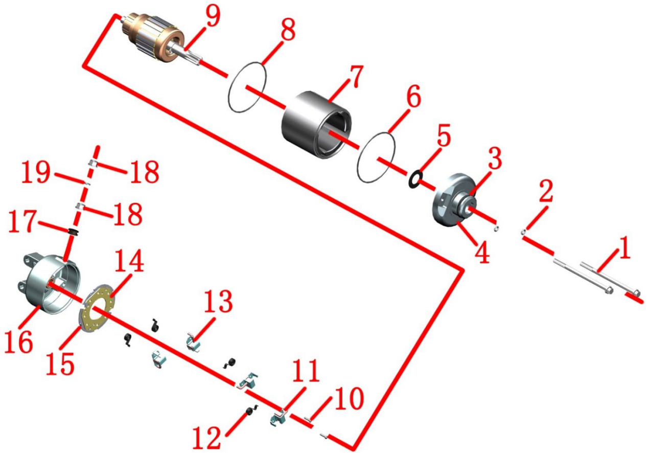
1-M6×90 螺栓×2 2-O 环×2 3-O 环 4-起动电机前盖 5-垫片 6-矩形密封圈 7-起动电机外过壳 8-矩形密封圈 9-电枢 10-螺钉×2 11-负极电刷×2 12-蜗簧×4 13-正极电刷×2 14-刷机架 15-刷机架绝缘垫片 16-起动电机后盖 17-绝缘垫 18-螺母×2 19-垫片
