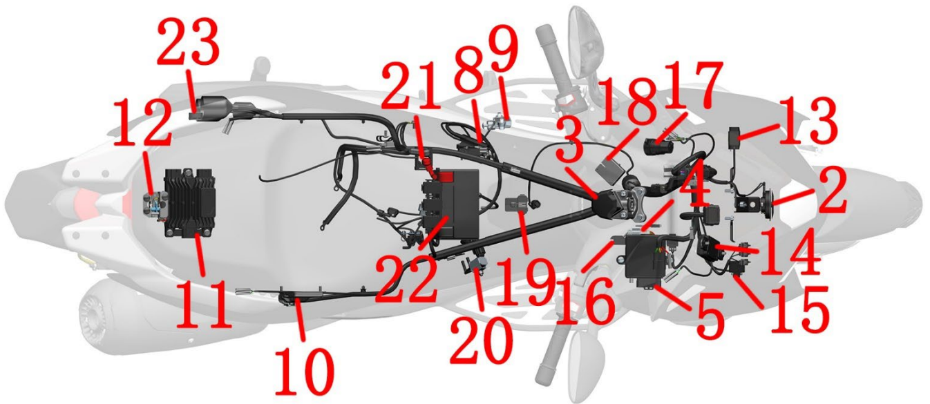
1-TFT 仪表 2-喇叭 3-龙头锁 4-充电口座 5-PKE 6-主电缆 7-GPS 天线 8-电喷高压线 9-侧支架熄火开关 10-发动机控制器 (ECU) 11-启停控制器 12-坐垫锁 13-倾倒开关 14-风挡电机控制器 15-闪光器 16-感应天线 17-USB 充电线 18-前储物箱锁 19-电子油箱锁 20-碳罐电磁阀 21-启动继电器 22-蓄电池 23-PKE 蜂鸣器
