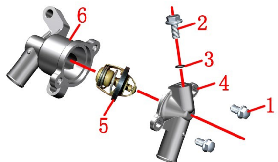
1-M6×10 螺栓*2 2-M6×12 螺栓 3-φ5.6×φ1 0 环 4-节温器上壳体 5-节温器芯体 6-节温器下壳体
