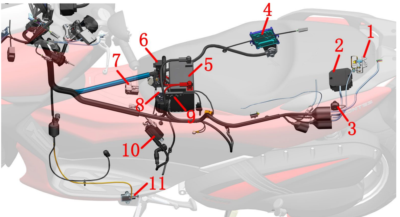
1-坐垫锁 2-整流器 3-蜂鸣器 4-发动机控制器 (ECU) 5-蓄电池 6-保险盒 7-电子油箱锁 8-保险盒 9-保险盒 10-点火线圈 11-侧支架熄火开关
