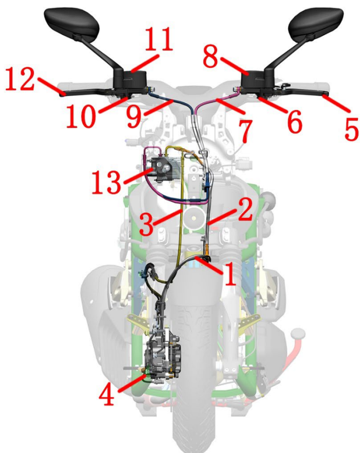
1-轮速传感器（前轮） 2-FC-HU 制动软管 3-RC-HU 制动软管 4-轮速传感器（后轮） 5-后制动手柄 6-后刹车开关 7-RMC-HU 制动软管 8-后碟刹主泵 9-FMC-HU 制动软管 10-前刹车开关 11-前碟刹主泵 12-前制动手柄 13-液控单元
