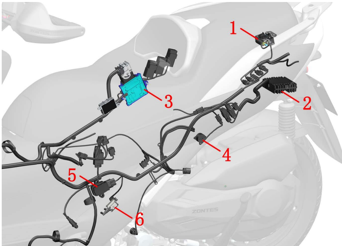
1-坐垫锁 2-整流器 3-发动机控制器 (ECU) 4-蜂鸣器 5-点火线圈本体 6-碳罐电磁阀
