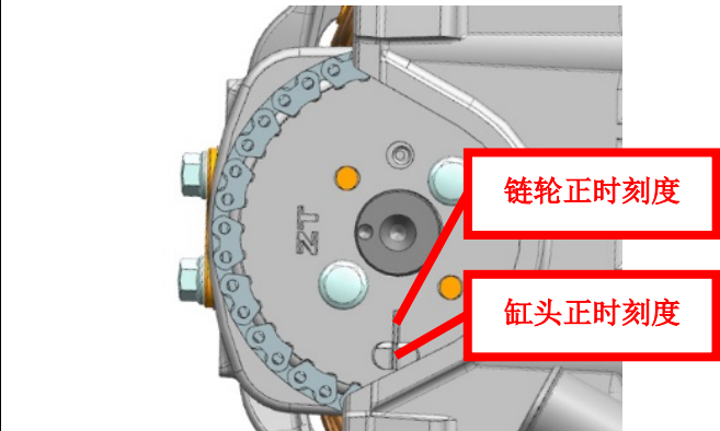
链轮正时刻度与缸头正时刻度对齐 飞轮检具：
