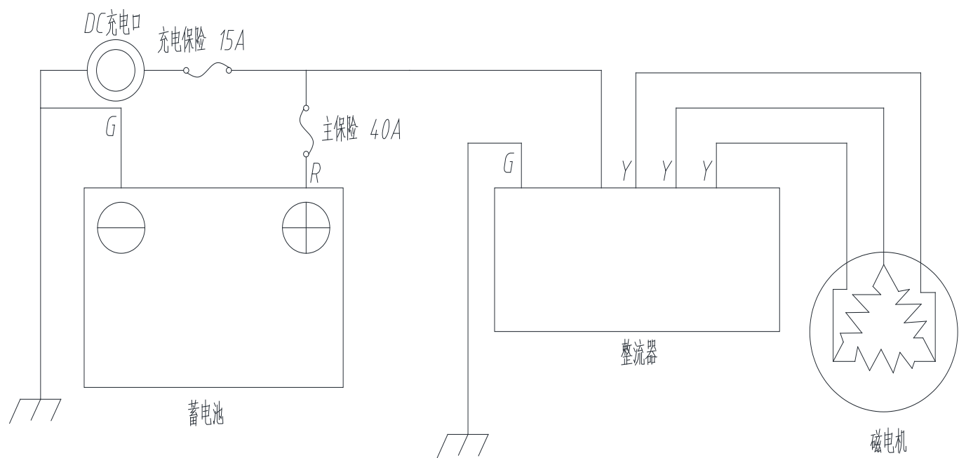
电气原理图
