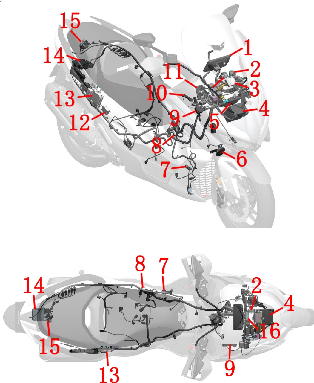
1-TFT 仪表 2-闪光器 3-智能控制盒 4-蓄电池 5- PKE 6-喇叭 7-侧支架熄火开关 8-碳罐电磁阀 9- GPS 天线 10-无电感应天线 11-龙头锁 12-胎压接收主机 13-发动机控制器 (ECU) 14-整流器 15-坐垫锁 16-倾倒开关
