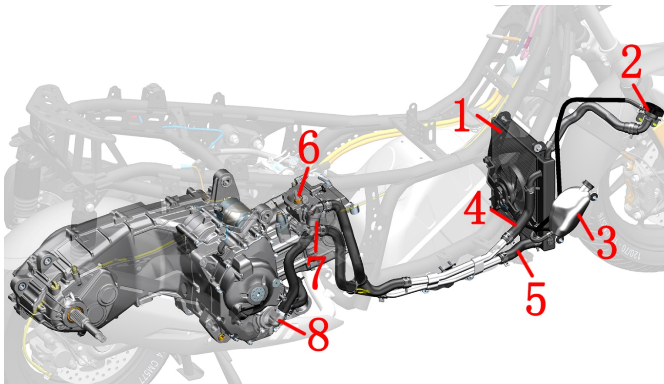
冷却系统分布图
