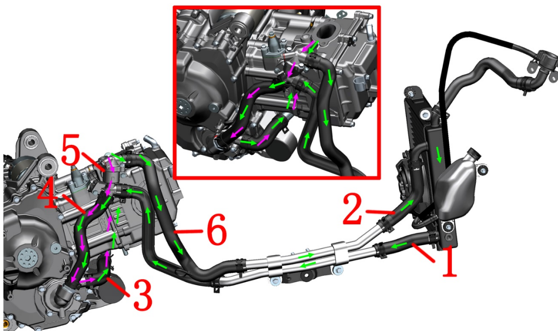
1-主水箱出水管 2-主水箱进水管 3-水泵盖出水管 4-水泵盖进水管 5-节温器 6-节温器出水管
