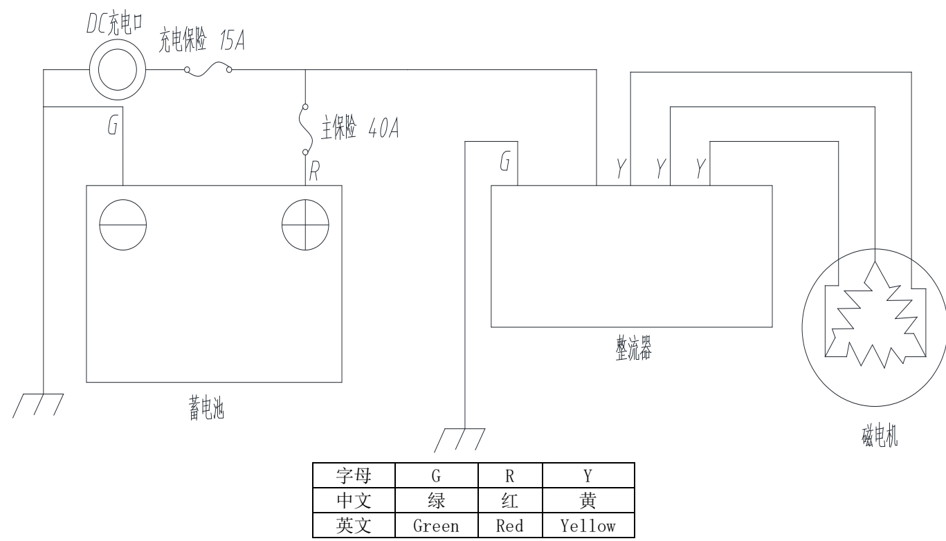
电气原理图
