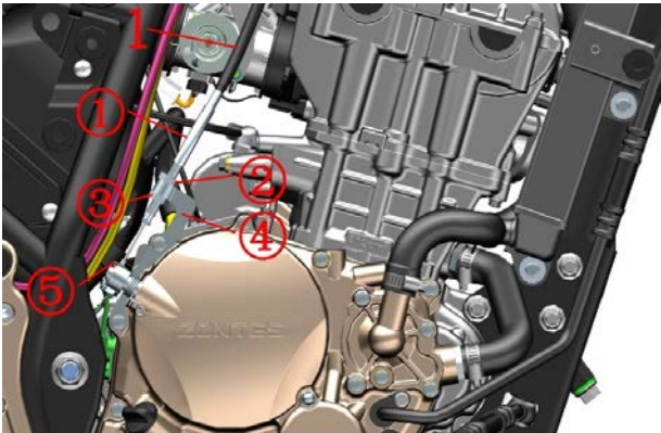
ZT310-R1离合线
