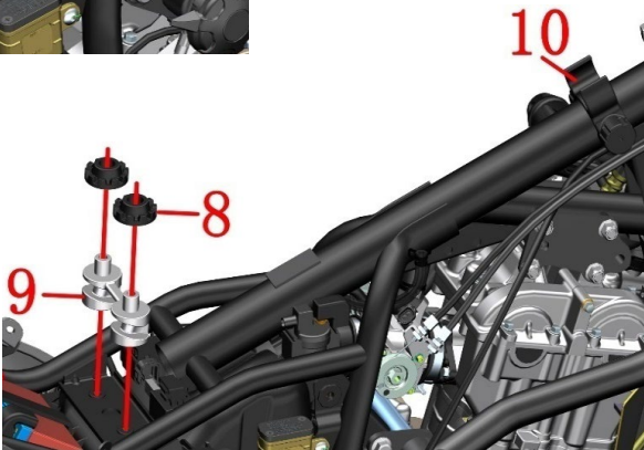
油箱锁插头
