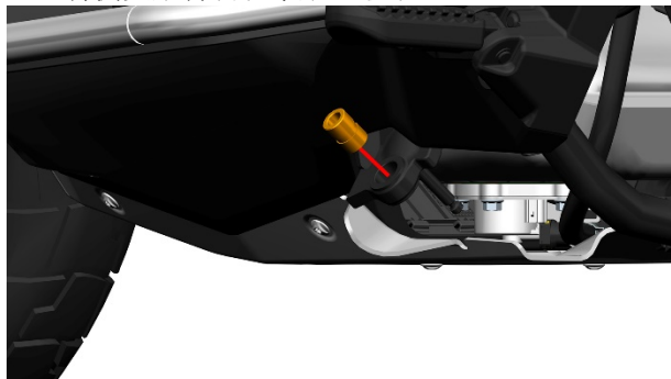
g. 使用柴油或煤油，或者干净的抹布将残留的润滑脂擦拭干净。在侧支架内侧 2 个安装平面、衬套外表面涂抹适量润滑脂，尽量不要涂抹到螺纹孔内。
