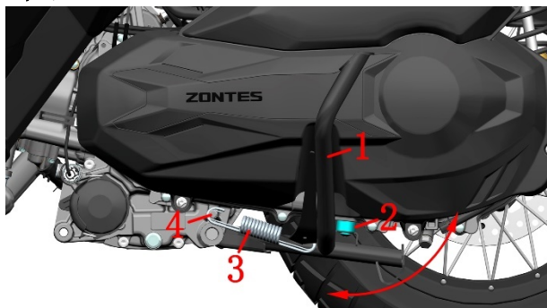
1. 主支架 2. 缓冲胶 3. 主支架弹簧 4. 主支架复位弹簧柱
