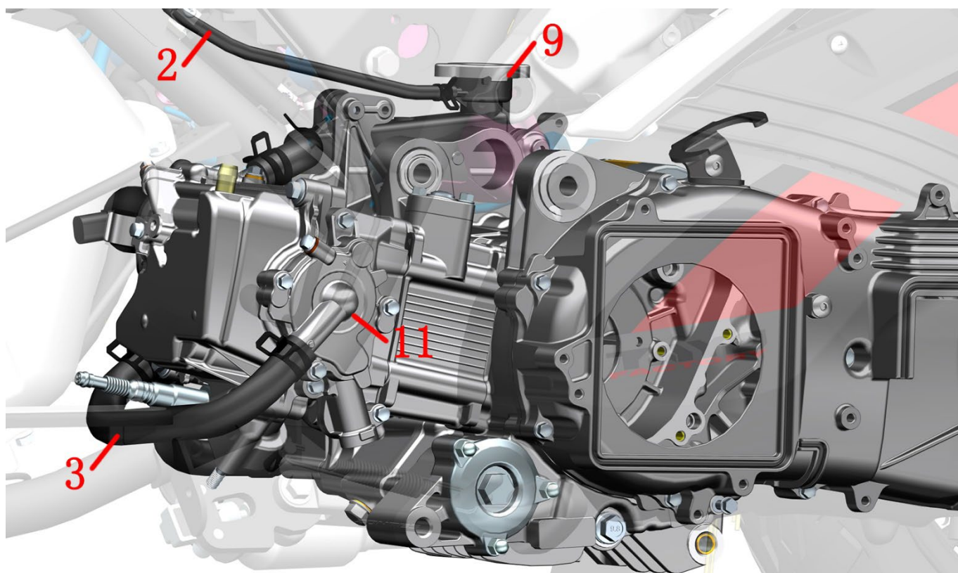
1-副水箱 2-副水箱连接水管 3-发动机进水管 4- 节温器出水管 5- 节温器 6- 水箱进水管 7- 水油共用传感器 8- 水箱出水管 9- 水箱盖(不可打开, 副水箱有冷却液时会从此处漏出) 10- 水箱 11- 水泵盖
