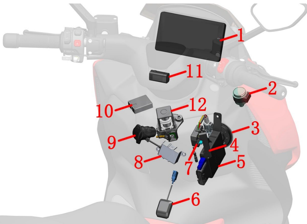
1-TFT 仪表 2-闪光器 3-喇叭 4-无电感应天线 5-PKE 6-GPS 天线 7-充电口座 8-胎压主机 9-USB 充电线 10-前储物箱 锁 11-倾倒开关 12-龙头锁
