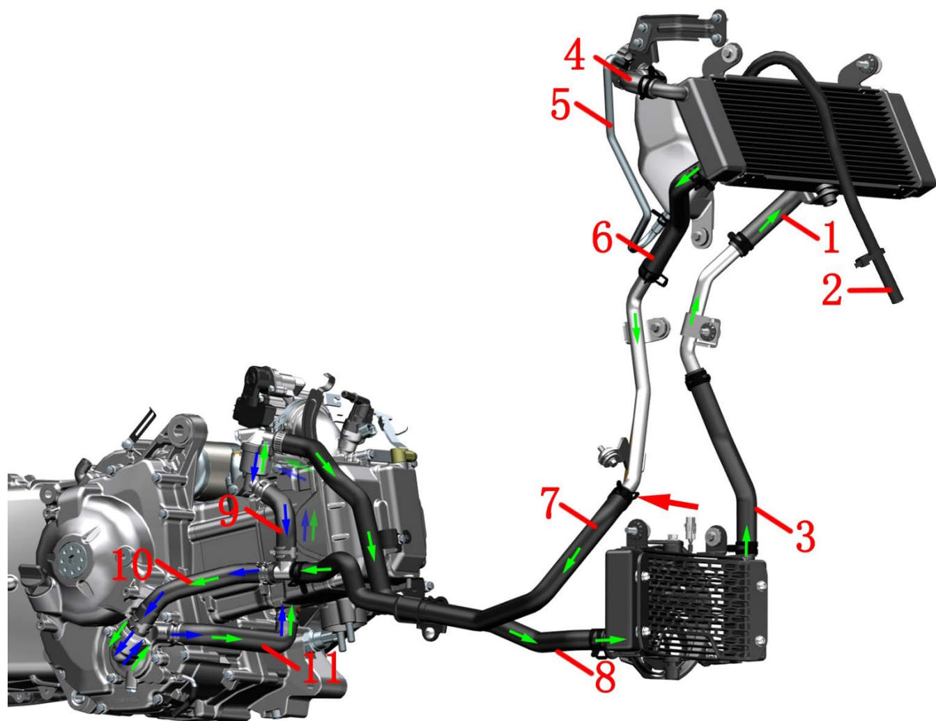
1-主水箱进水管 2-漏水管 3-小水箱出水管 4-加水口水管 5-副水箱连接水管 6-主水箱出水管 7-发动机进水管 8-小水箱进水管 9-小循环出水管 10-水泵盖进水管 11-气缸进水管
