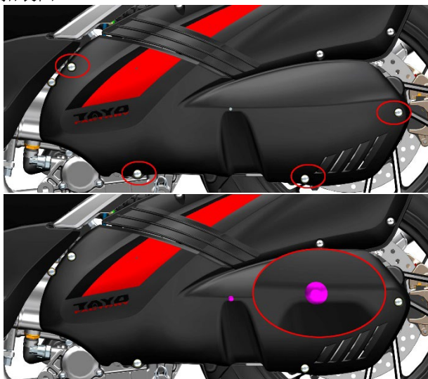
g. 用 4# 内六角将另外 4 颗 M6×14 轴肩内六角螺栓或 T30 梅花扳手将 4 件小法兰 M6×16+衬套+胶垫装回。将装饰扣装回。
