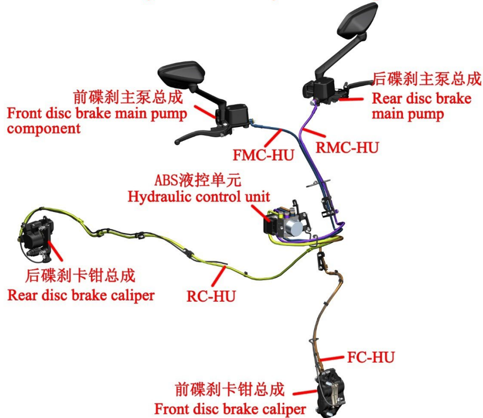
制动系统总成示意图 Brake system assembly sketch map
