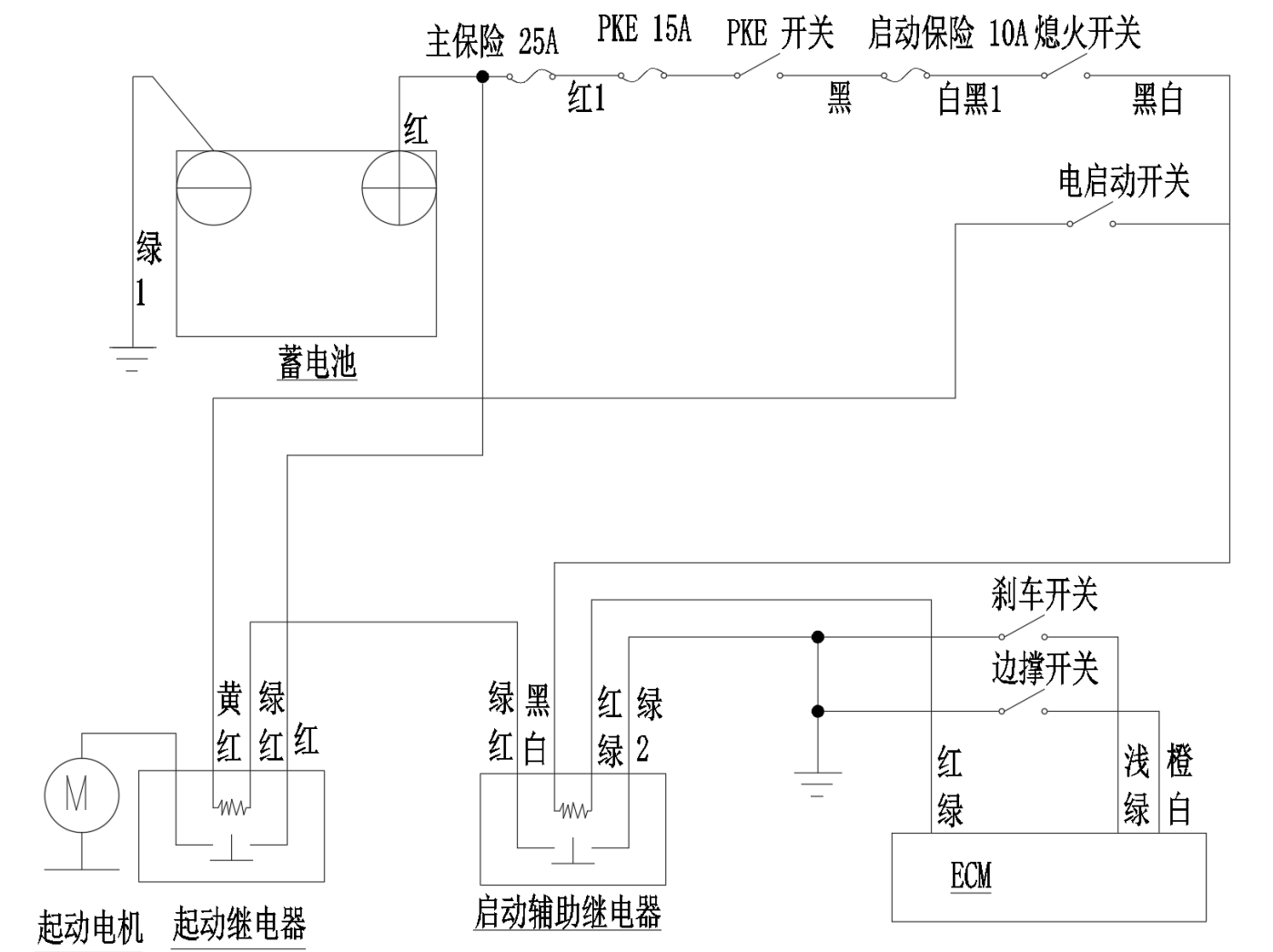
起动系统电气原理图 D350/368
