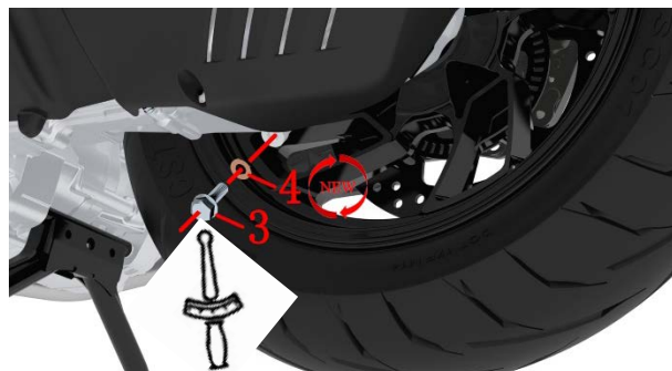
c. 将 M8×25 放油螺栓(3)和 8.3×16×1.5 铜垫(4)取下。
