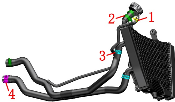
冷却液系统抱箍/卡箍分布图 D368/350
