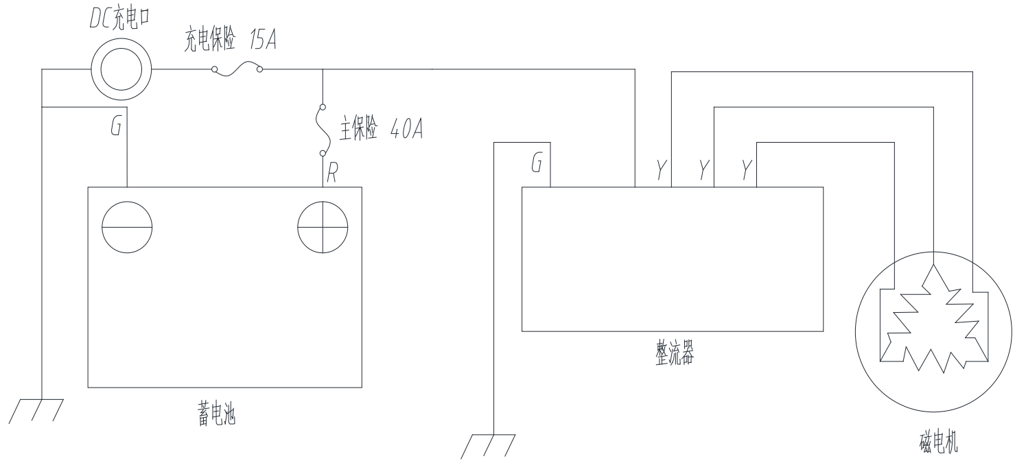
电气原理图
