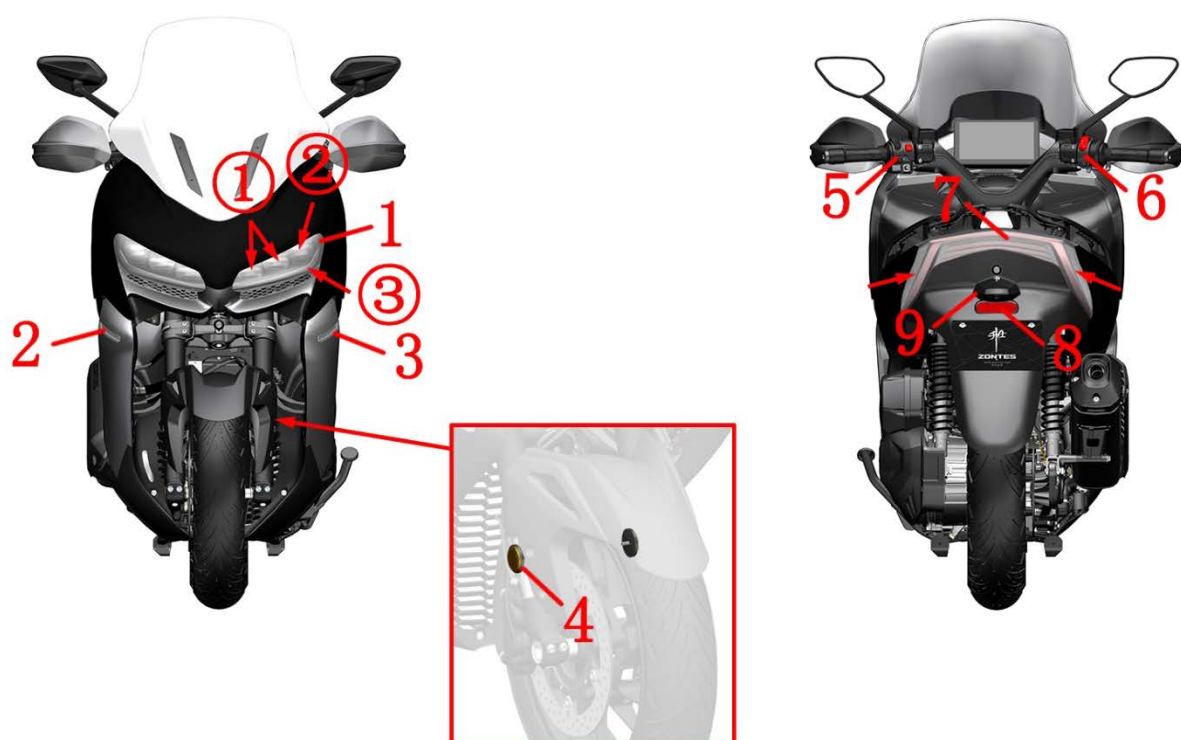
1-大灯 (①-近光灯位置 ②-远光灯位置 ③-位置灯/日行灯位置) 2-右转向灯 3-左转向灯 4-侧反射器 5-左手把开关 6-右手把开关 7-后尾灯 (④-后左转向灯 ⑤-后右转向灯) 8-后反射器 9-后牌照灯
