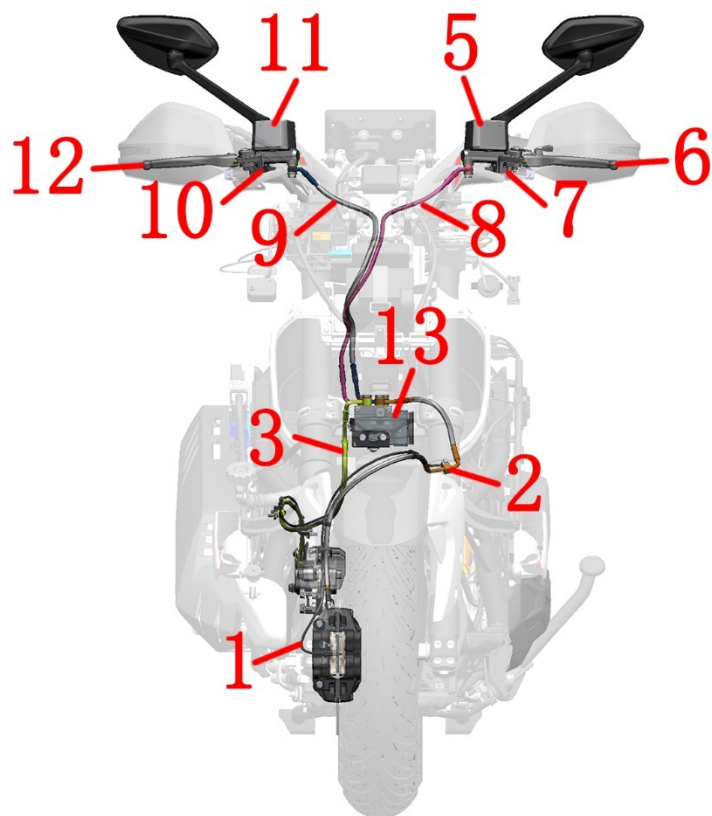
1-轮速传感器（前轮） 2-FC-HU 制动软管 3-RC-HU 制动软管 4-轮速传感器（后轮） 5-后碟刹主泵 6-后制动手柄 7-后 刹车开关 8-RMC-HU 制动软管 9-FMC-HU 制动软管 10-前刹车开关 11-前碟刹主泵 12-前制动手柄 13-液控单元
