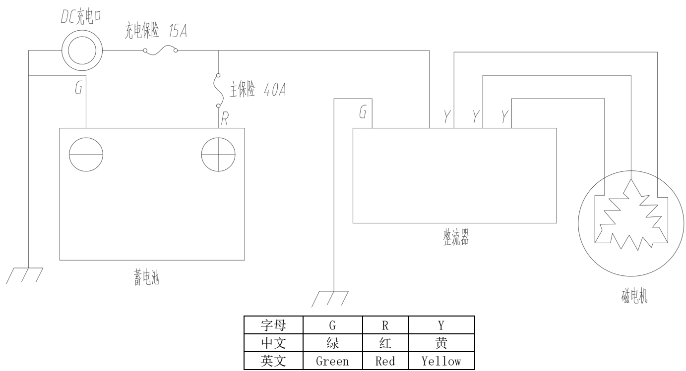
电气原理图
