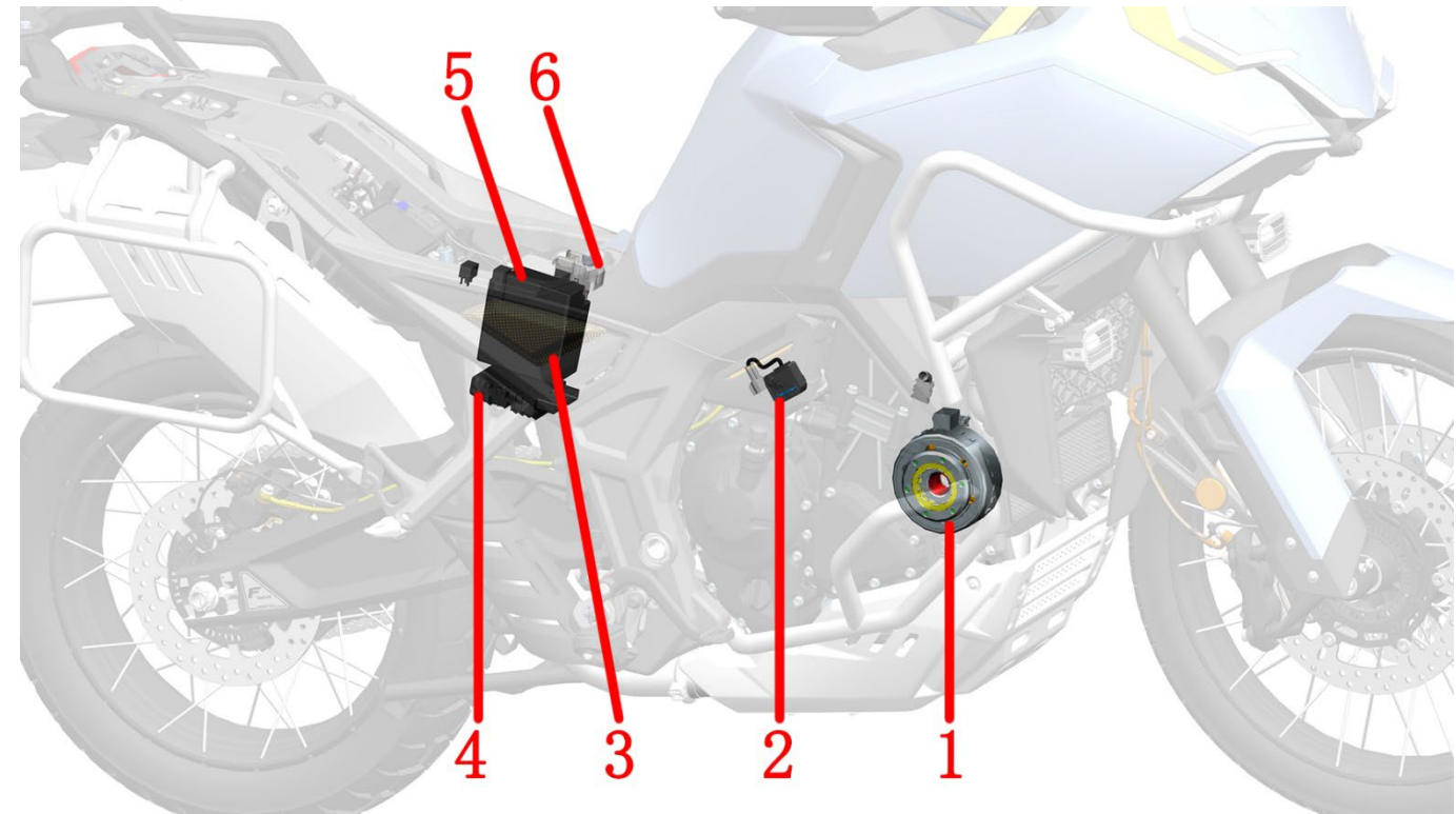
1-磁电机 2-充电口座 3-蓄电池 4-整流器 5-保险盒 6-启动继电器（40A）
