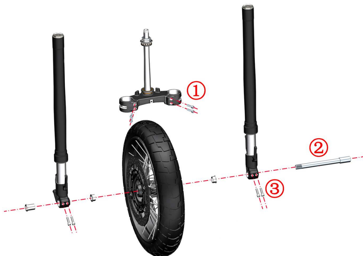
前叉分解图
