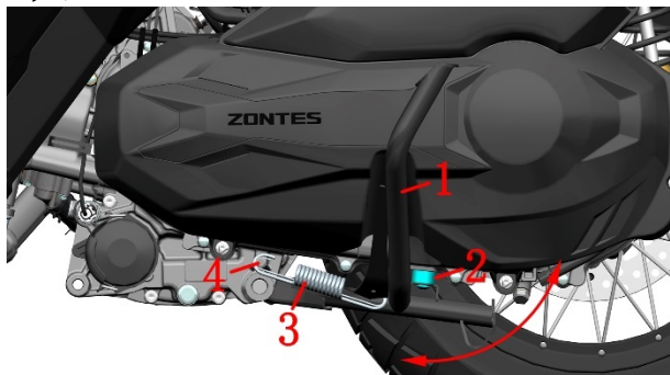
1. 主支架 2. 缓冲胶 3. 主支架弹簧 4. 主支架复位弹簧柱
