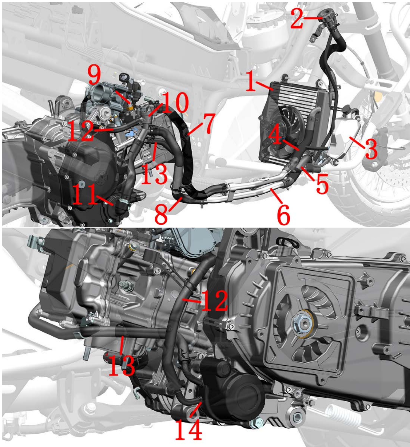
1-主水箱 2-水箱加水口 3-副水箱 4-主水箱进水管 5-主水箱出水管 6-铝过水管 7-节温器出水管 8-发动机进水管 9-水油共用传感器 10-节温器 11-水泵盖组件 12-油冷器进水管 13-油冷器出水管 14-油冷器
