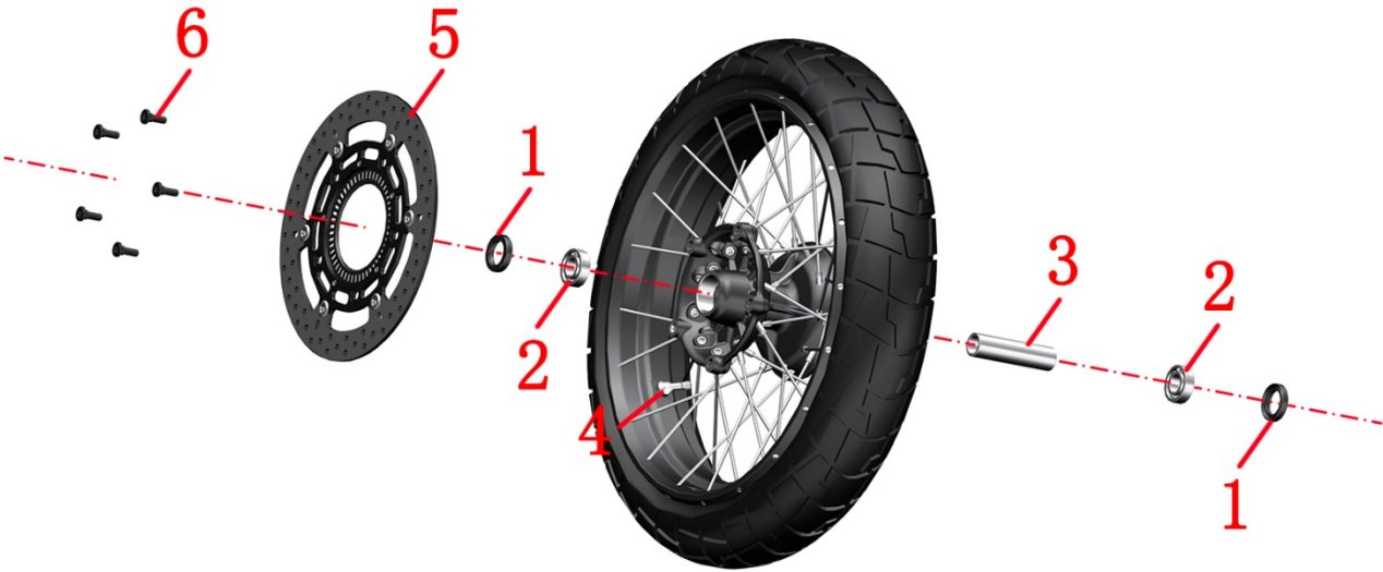
前轮组件分解图：
