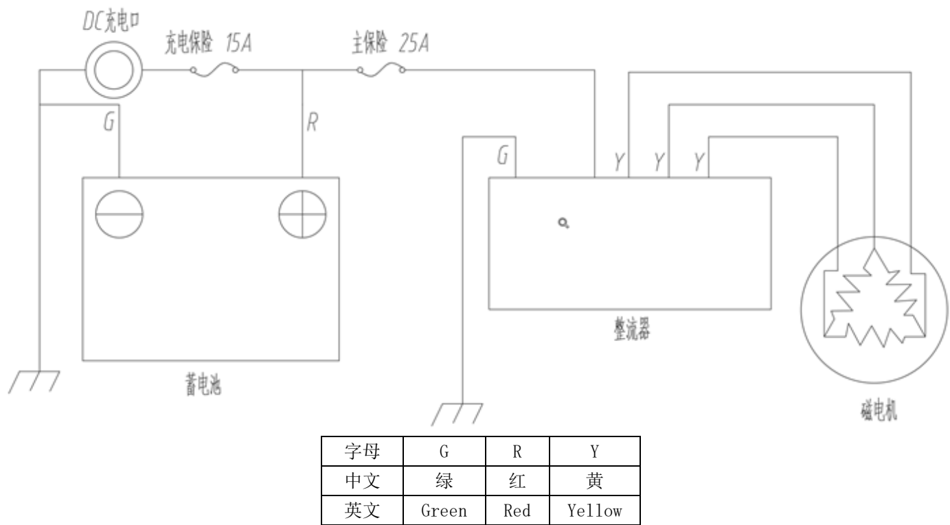
电气原理图
