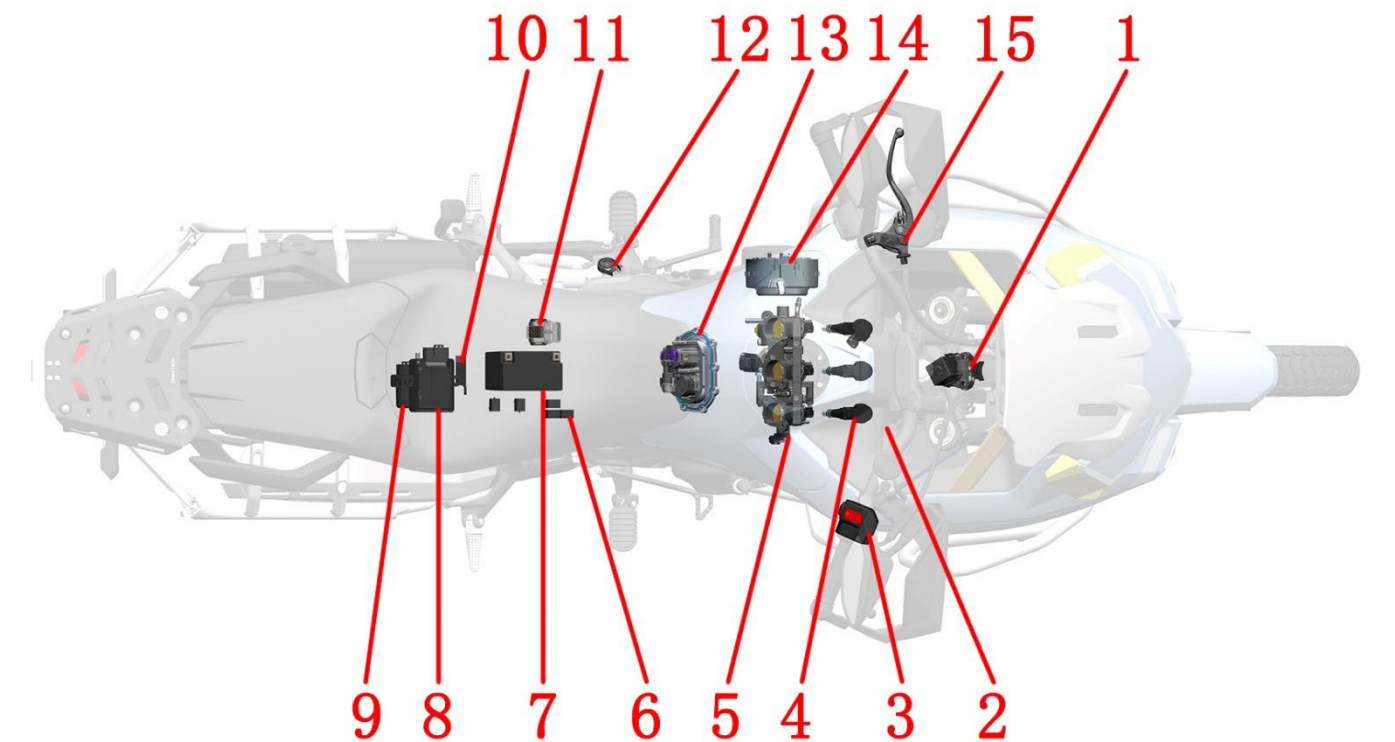
1-龙头锁 2-氧传感器 3-右手把开关 4-点火线圈 5-节气门组件 6-继电器（主线束保险盒内有3件，保险盒外侧有2件） 7-蓄电池 8-PKE 主机 9-ECU 10-倾倒开关 11-启动继电器 12-侧支架熄火开关 13-油泵泵 14-磁电机 15-离合摇臂
