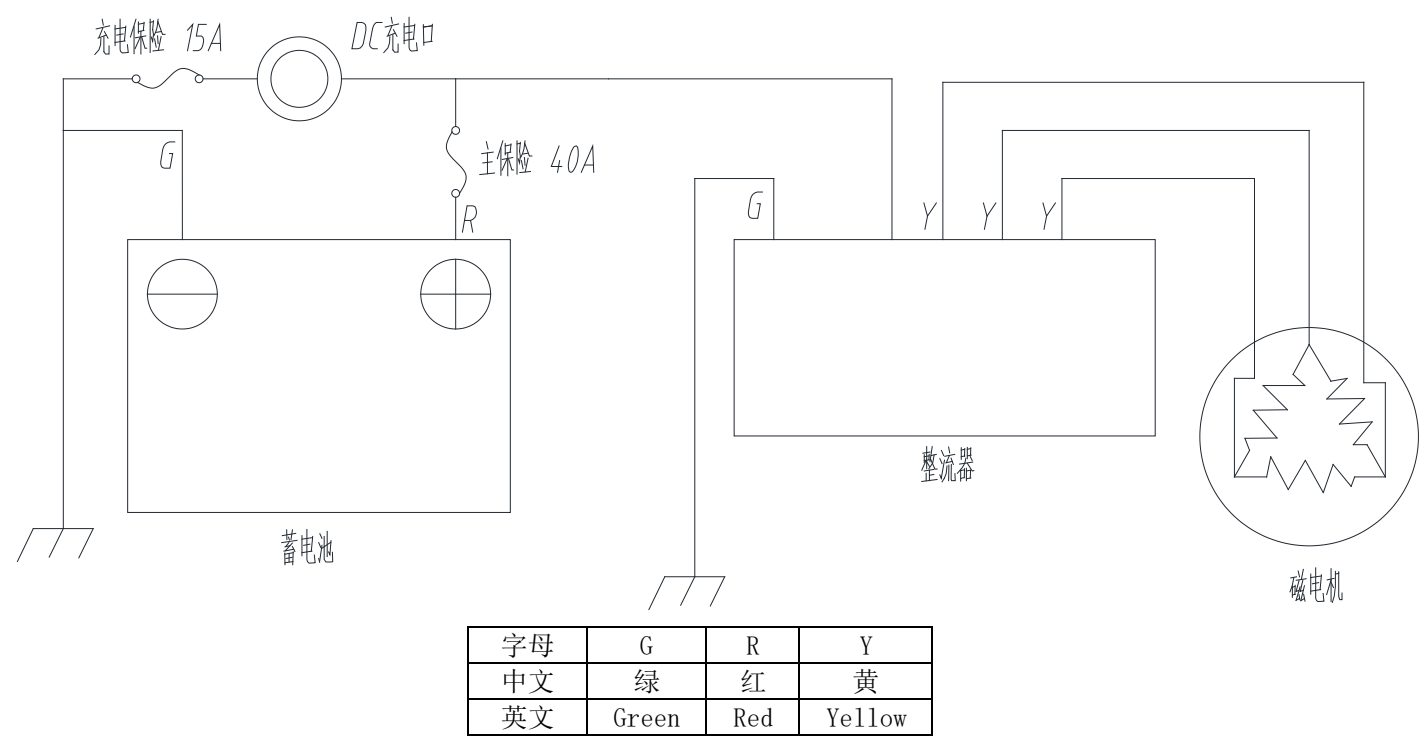
电气原理图
