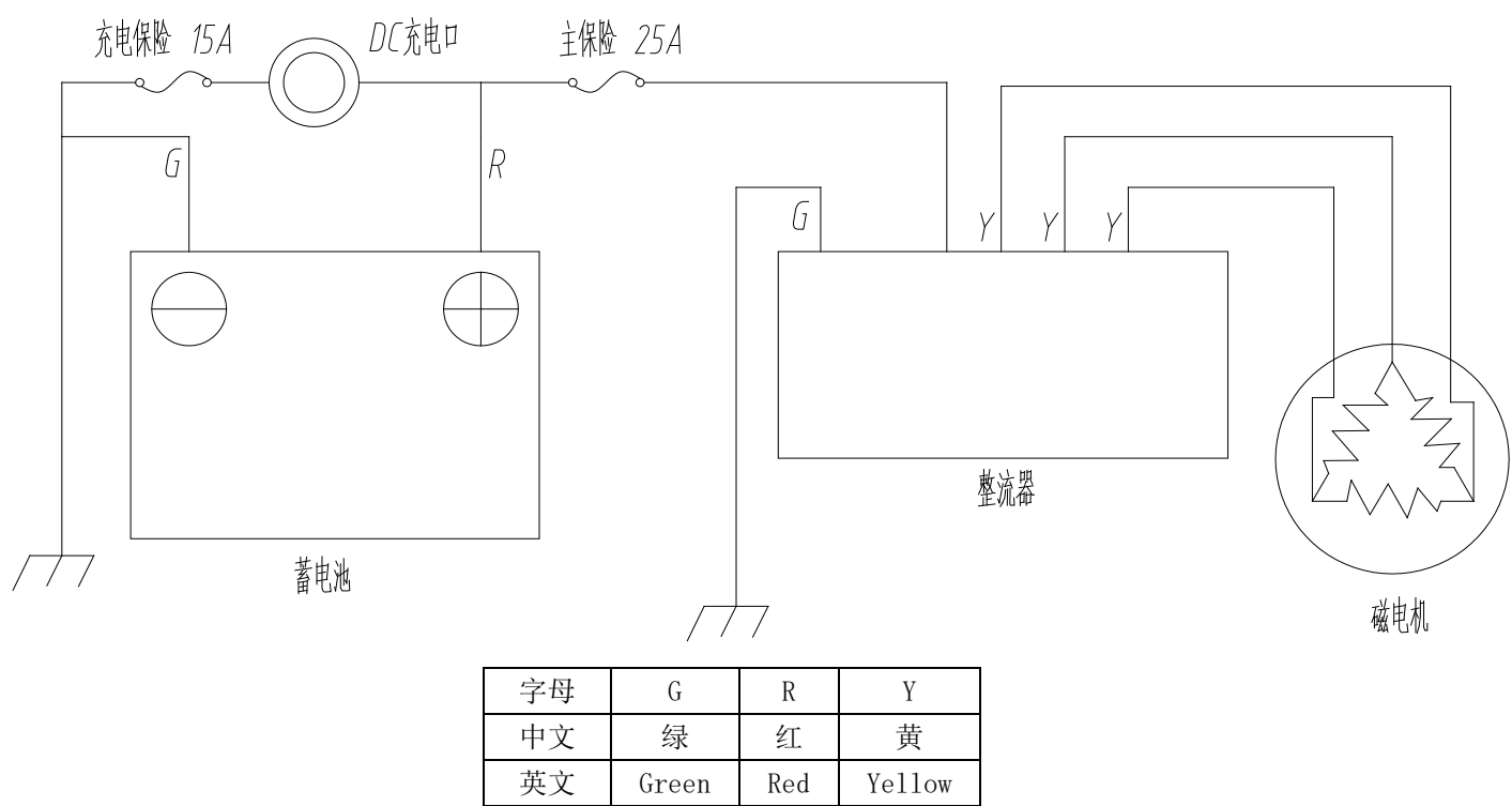
电气原理图
