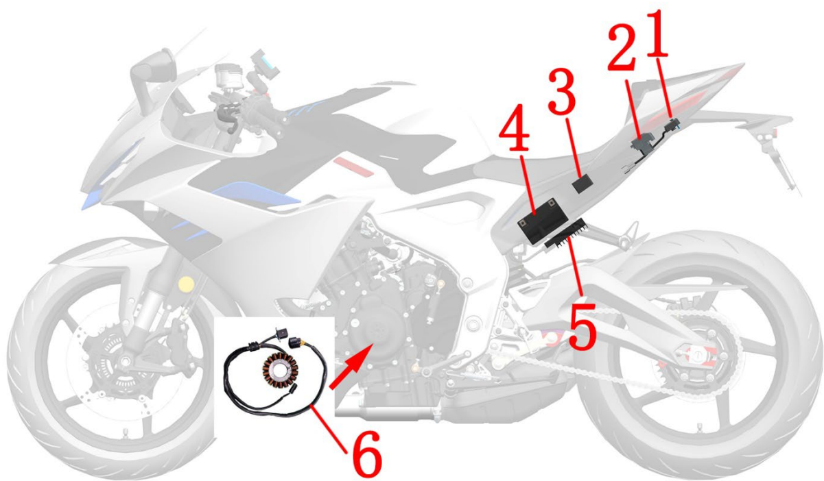
1-充电口座 2-启动继电器（40A）3-保险盒 4-蓄电池 5-整流器 6-磁电机
