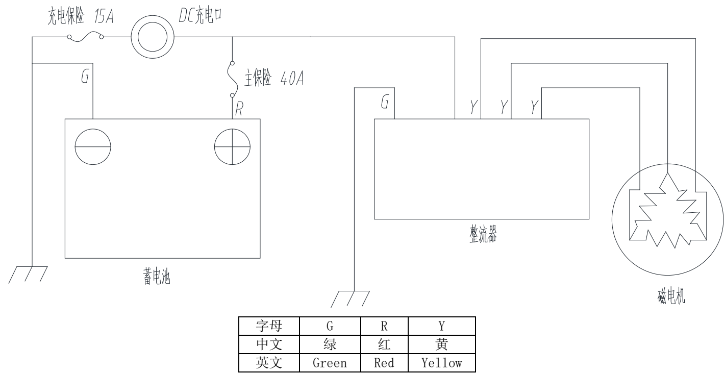
电气原理图
