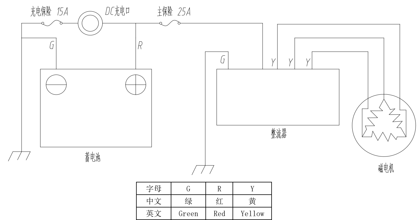
电气原理图
