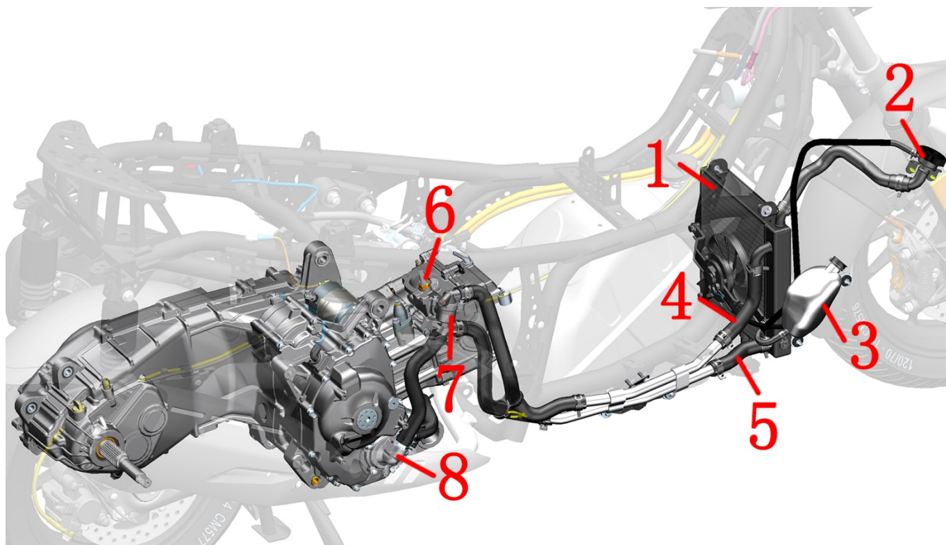
冷却液系统分布图
