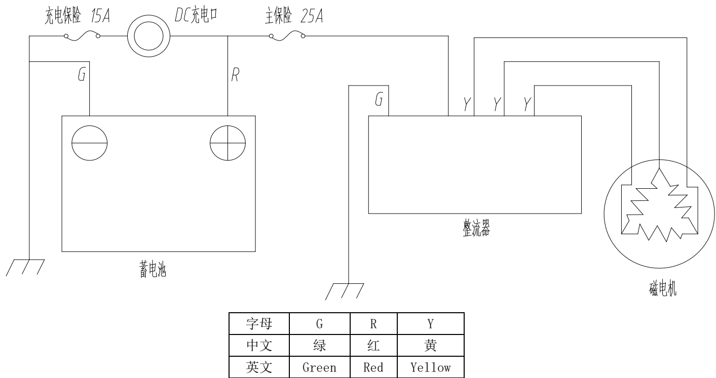
电气原理图
