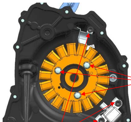
M5×15—5#内六角圆柱螺钉（氧化黑）
