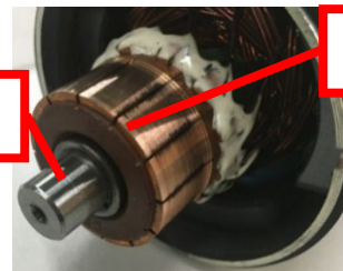
换向器
