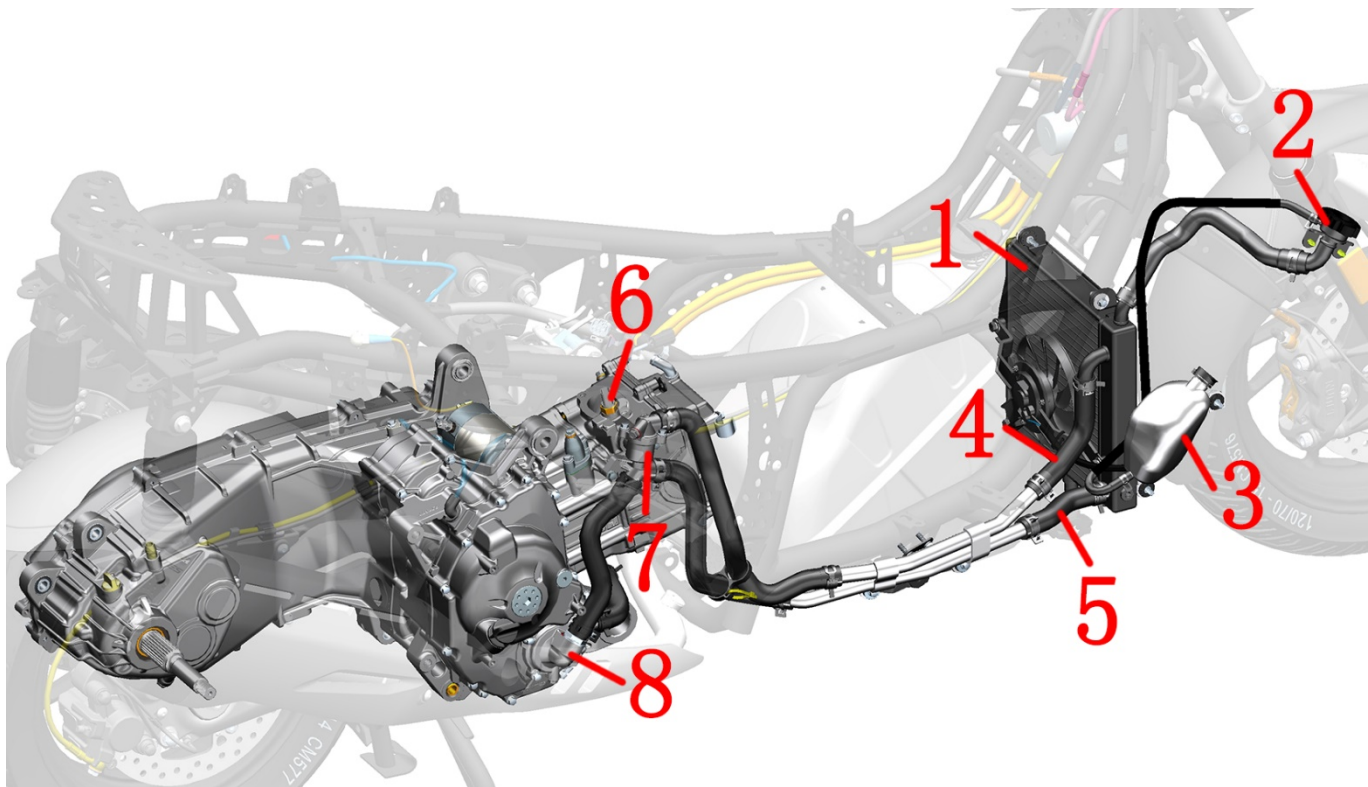
1-主水箱 2-水箱加水口 3-副水箱 4-主水箱进水管 5-主水箱出水管 6-水油共用传感器 7-节温器 8-水泵盖组件 冷却液流动示意图
