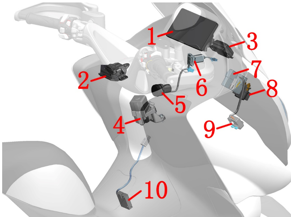
1-TFT 仪表 2-前左储物箱锁 3-风挡电机控制器 4-龙头锁 5- 双扣 USB 充电线 6-单口快充总成 7-电喷继电器 8-启动继电器 9-充电口座 10-油箱电子锁
