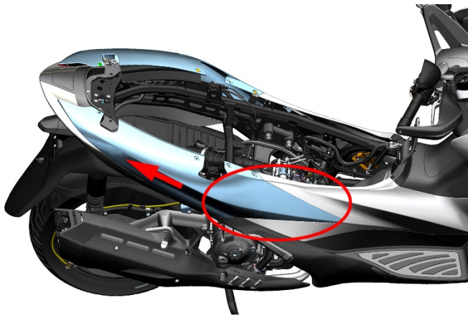
c. 左右后尾裙组件用同样方法拆装。
