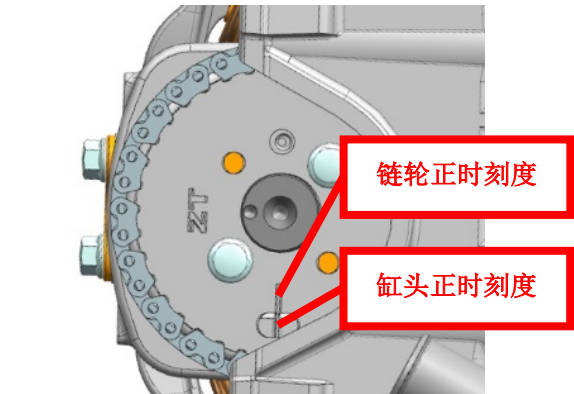
链轮正时刻度与缸头正时刻度对齐 飞轮检具：
