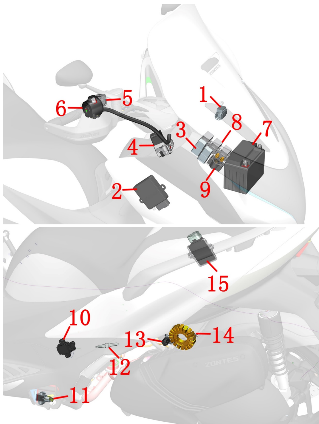
1-倾倒开关 2-PKE 3-继电器 4-龙头锁 5-右手把副开关 6-右手把开关 7-蓄电池 8-保险盒 9-启动继电器 10-点火线圈 11-侧支架熄火开关 12-火花塞 13-曲轴位置传感器 14-磁电机定子 15-ECU
