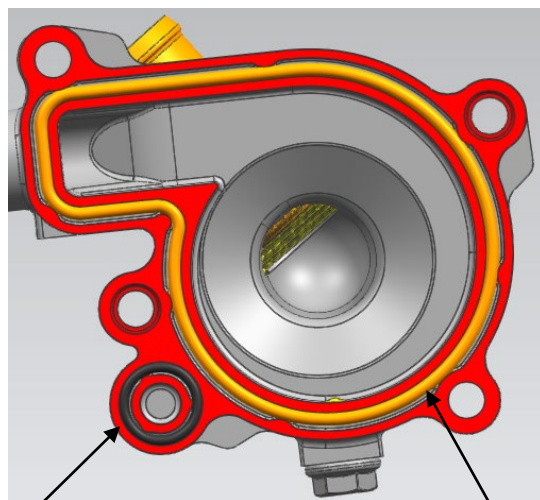
\phi 11.5 \times \phi 1.8 三元乙丙胶 O 型圈
