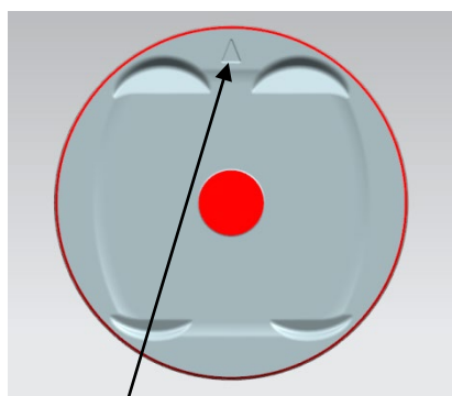
排气侧△标记
