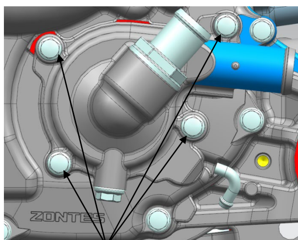
M6×30 六角法兰面螺栓
