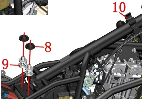
油箱锁插头
